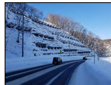
<対策例> 雪崩予防柵
