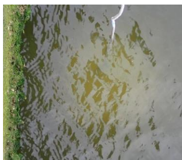
図2 海水の着色状況
