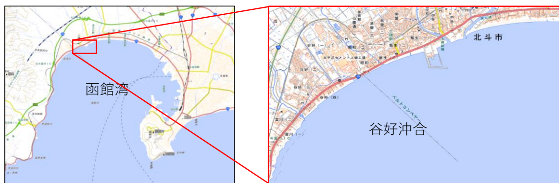
図1 赤潮発生場所の位置
