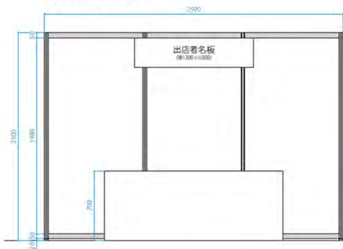
■ 立面図レイアウト(例)
