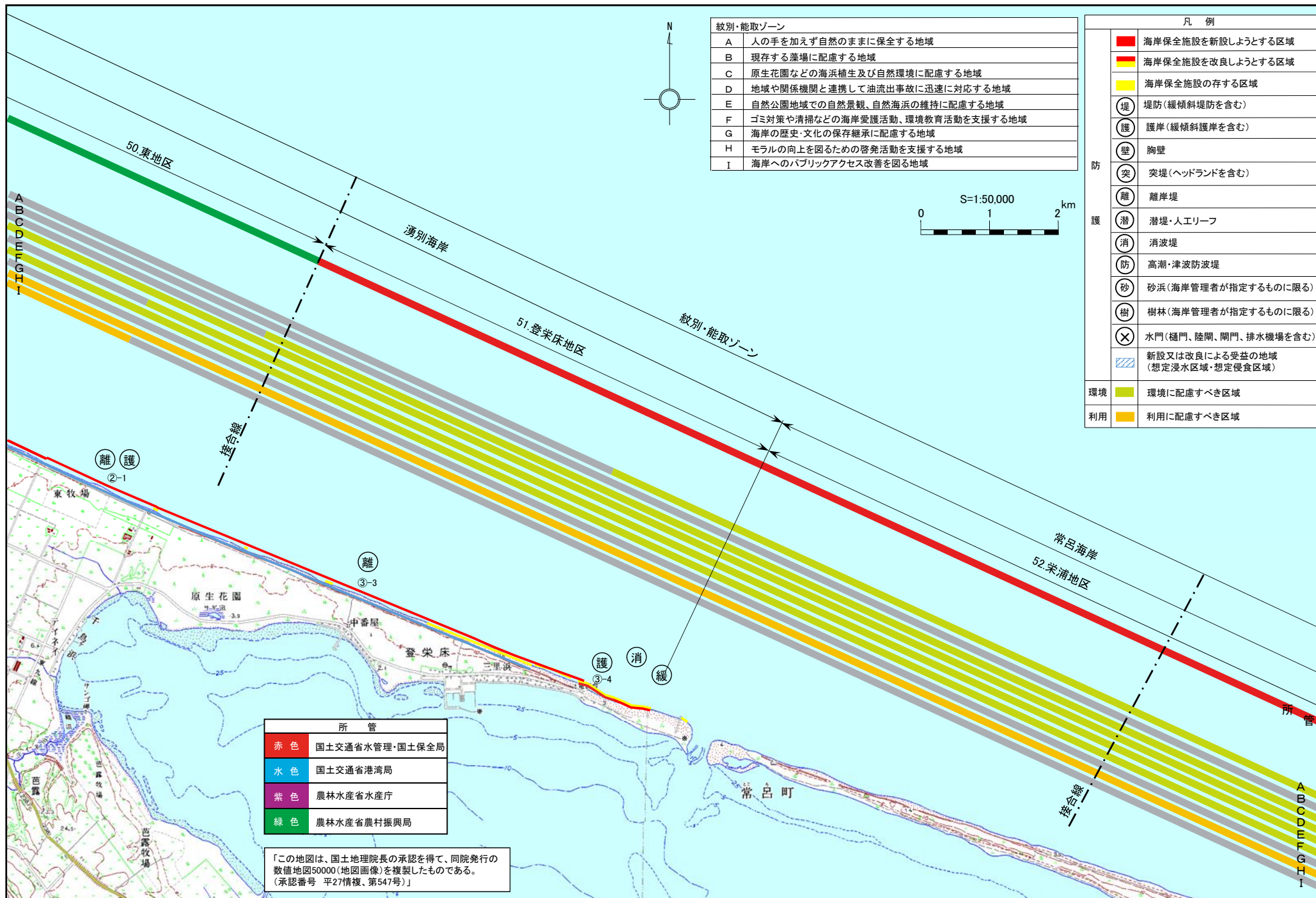
紋別・能取ゾーン 図面番号 4/7
