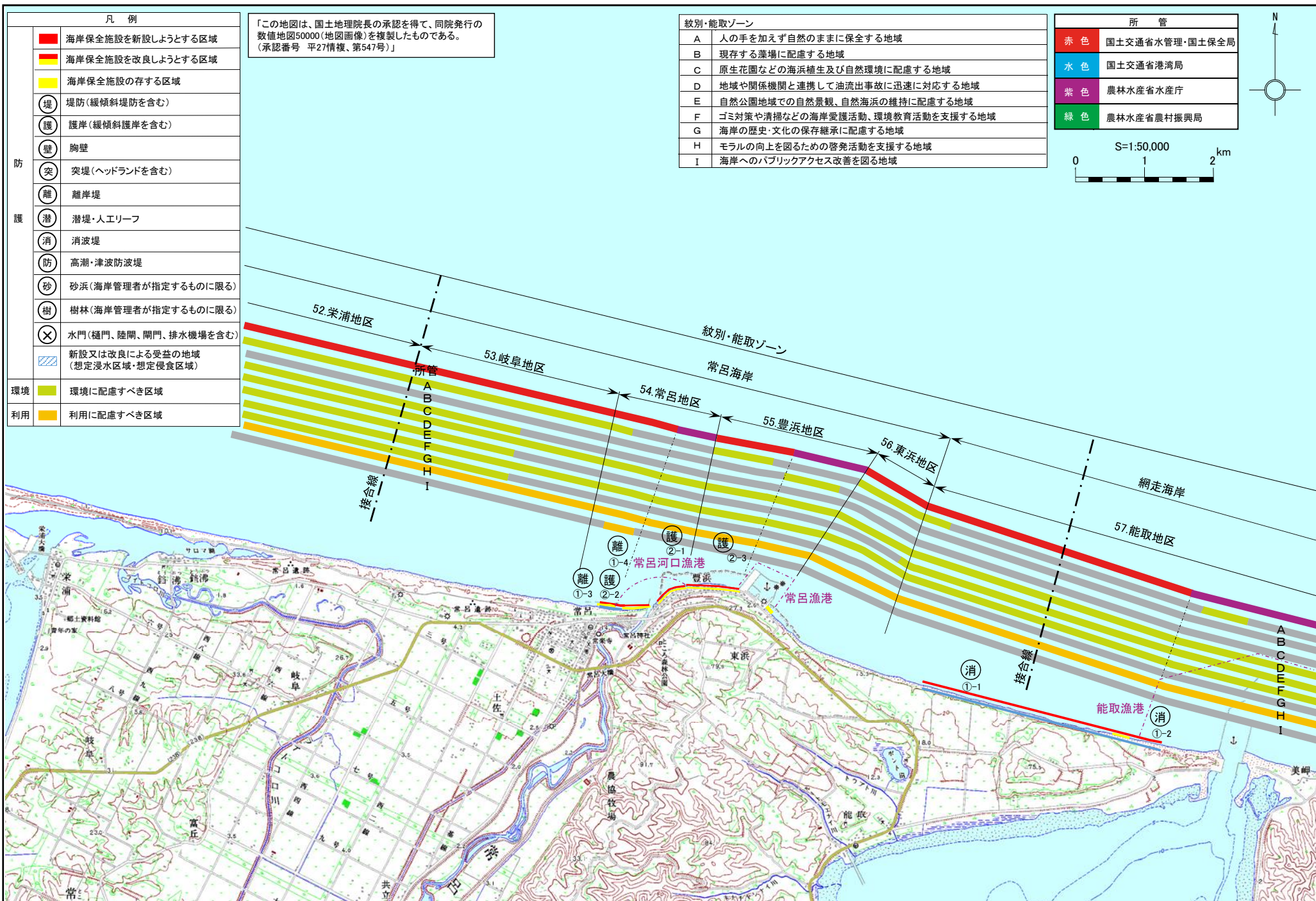
紋別・能取ゾーン 図面番号 6/7
