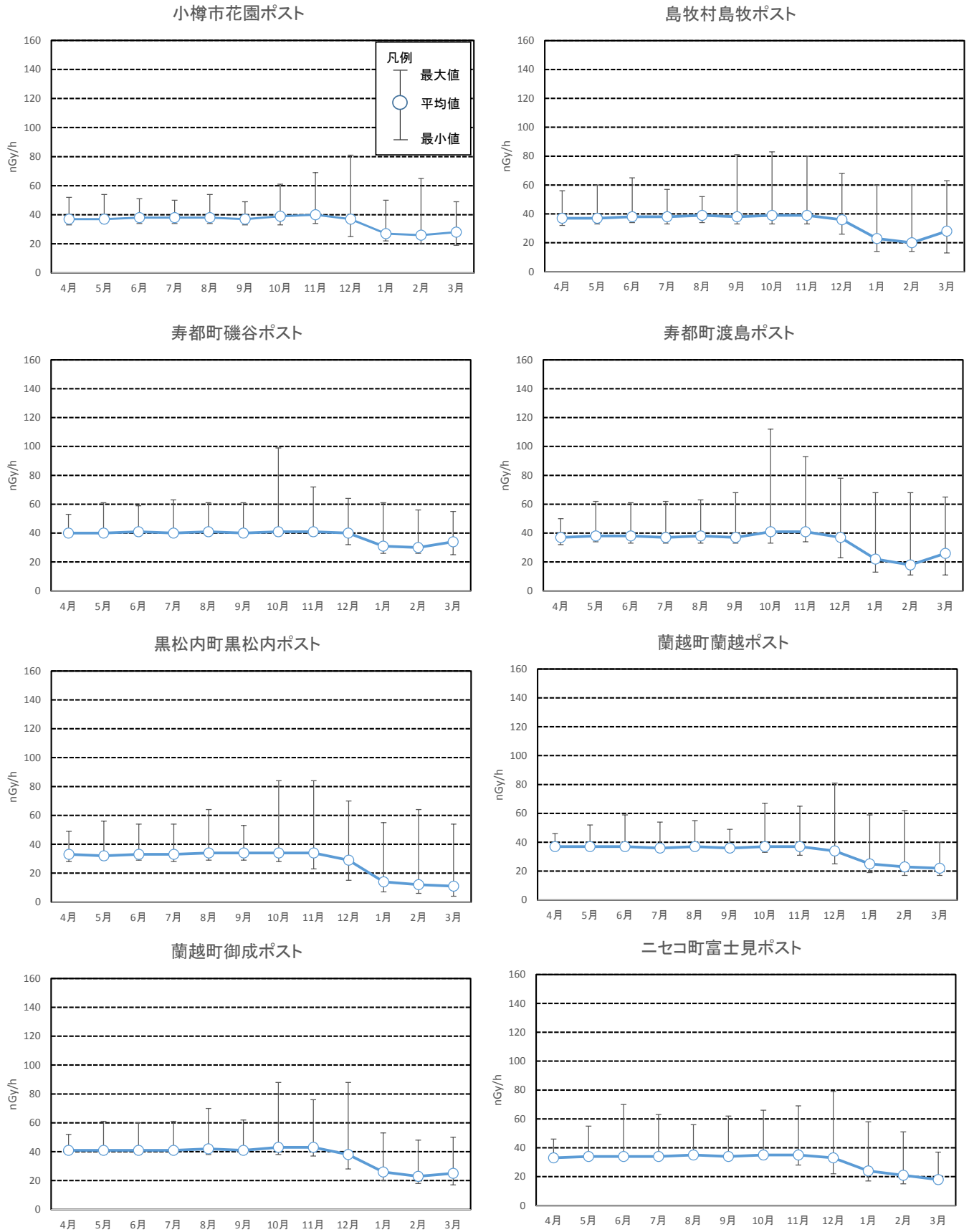
図3 空間放射線量率の経月変化図
