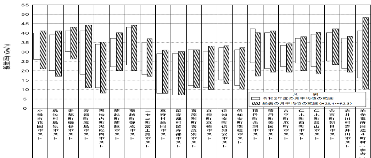
図2 各測定局の空間放射線量率の範囲（月平均値）
