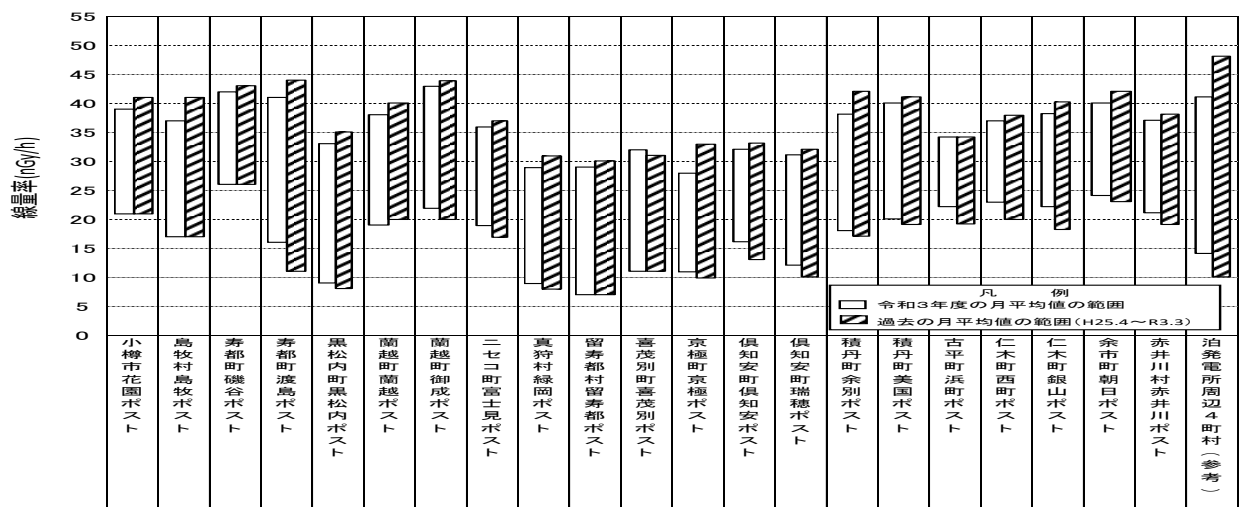
図2 各測定局の空間放射線量率の範囲（月平均値）
