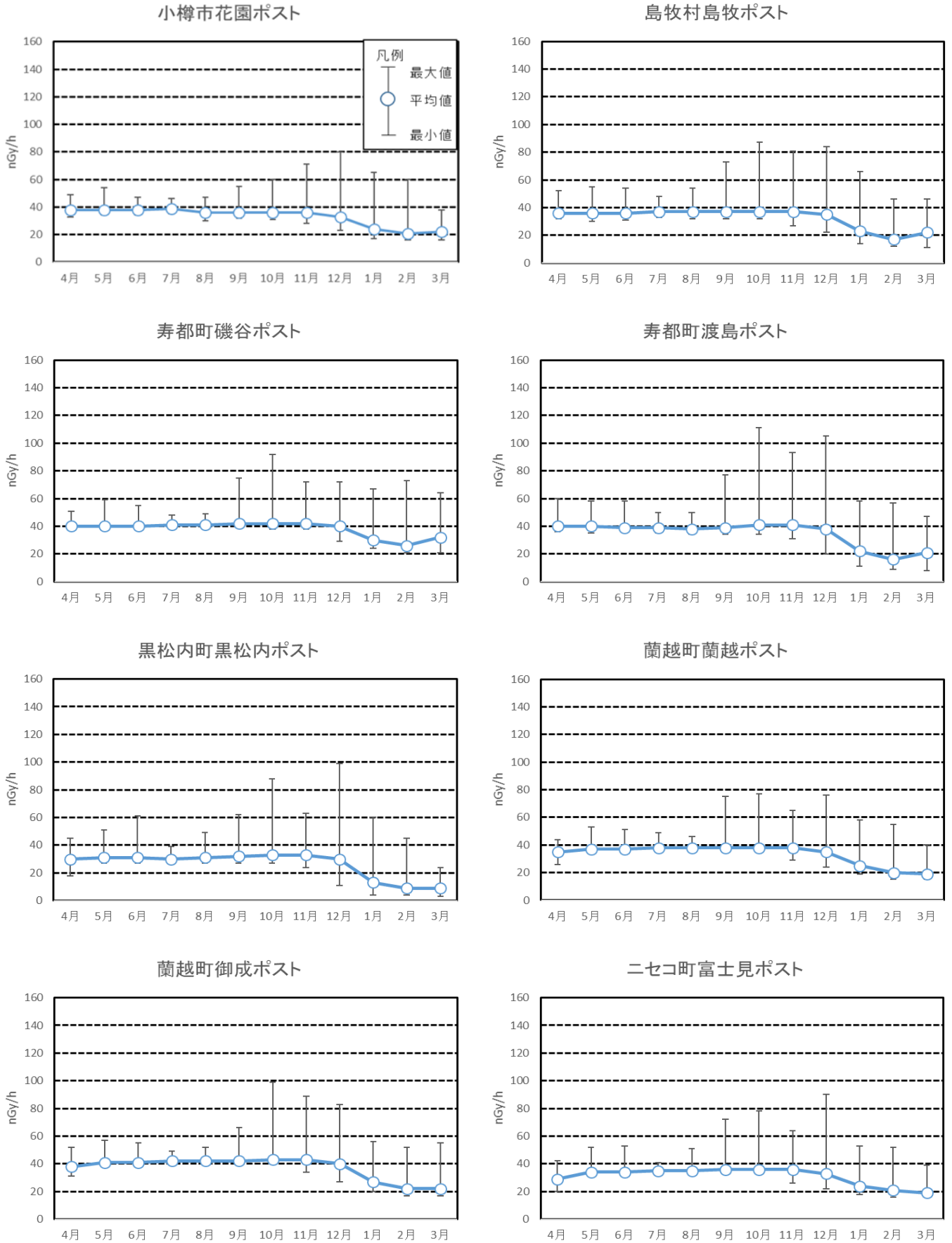
図3 空間放射線量率の経月変化図
