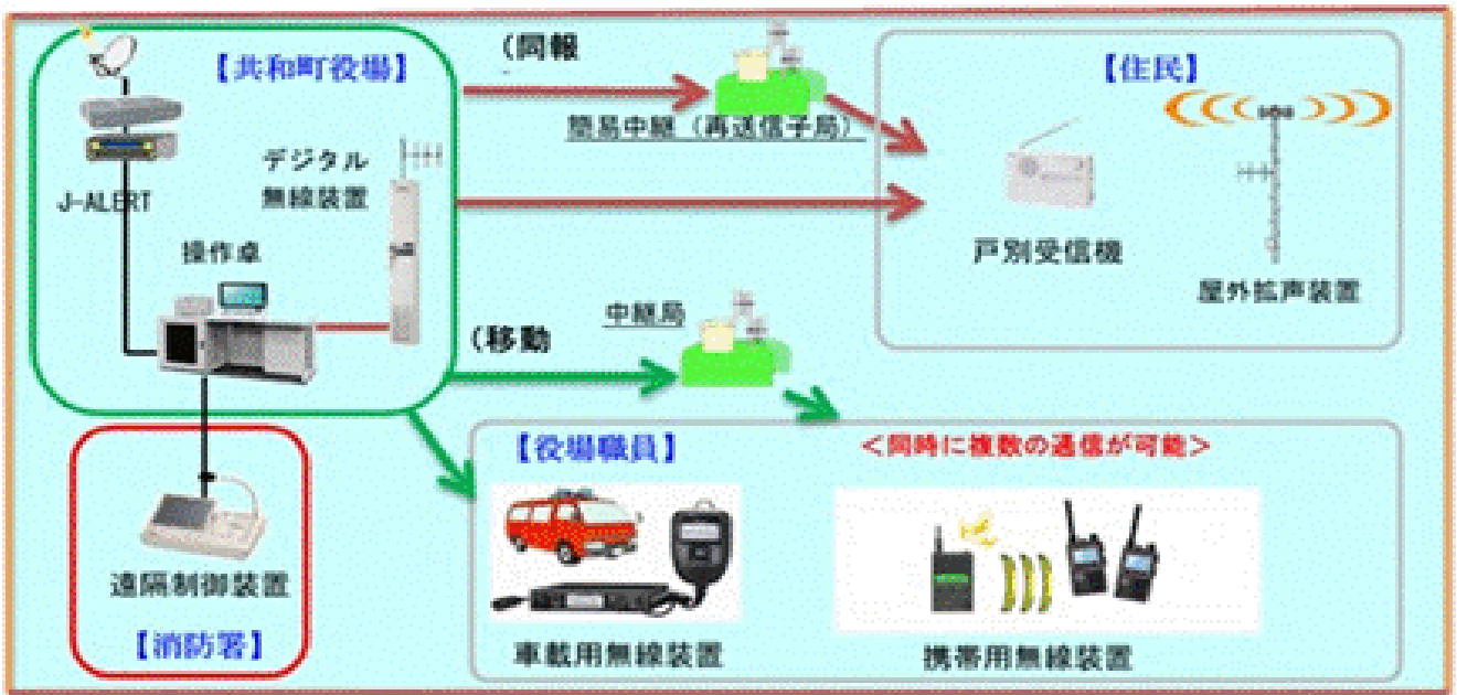
防災行政無線システム図
