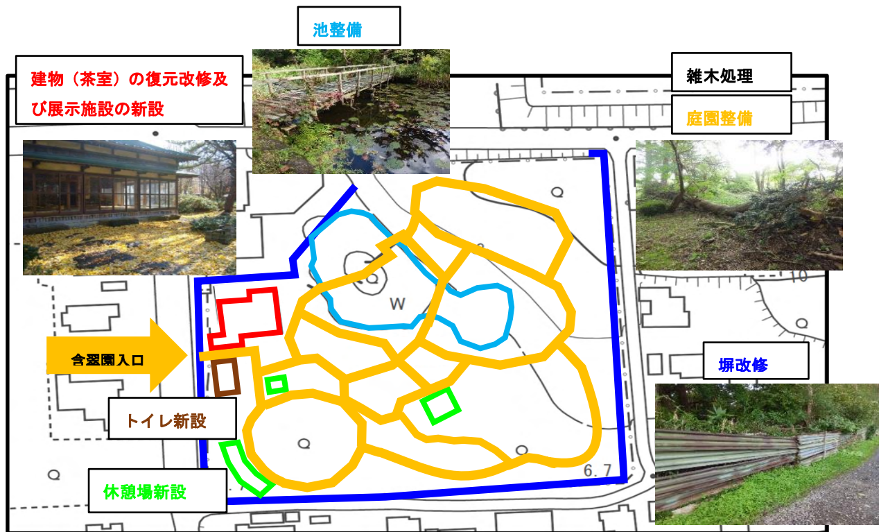
含翠園改修予定概要図
