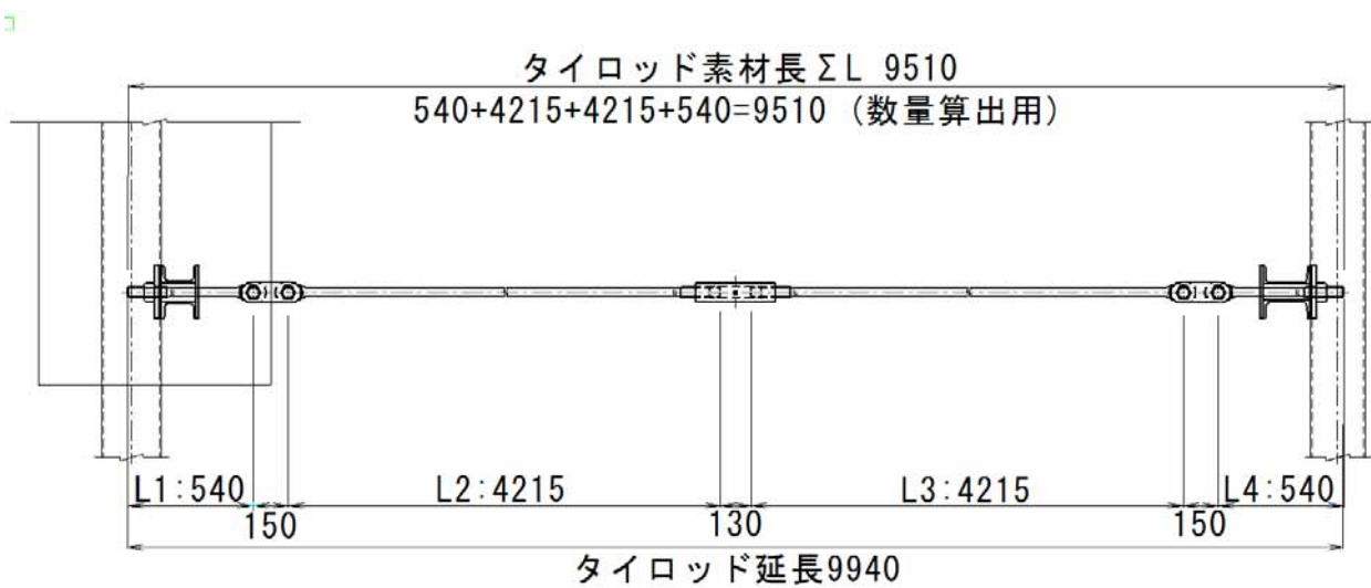
タイロッド素材長算定 (例)
