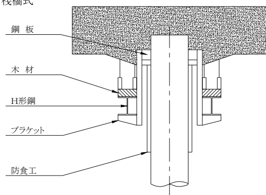
栈橋式
