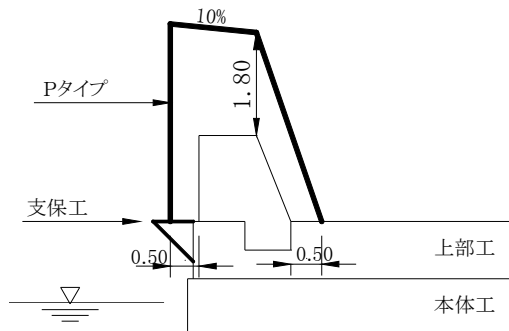
④ 胸壁コンクリート（構造物高さ h \leq 1.6\text{m} ）
