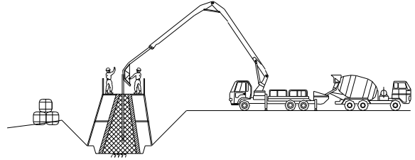
4) 本土工 場所打擁壁工 (構造物単位)
