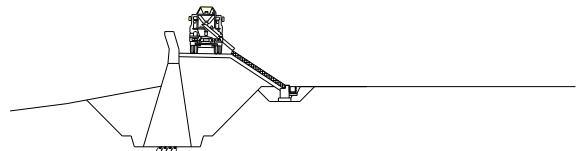
10) 裏法被覆工 コンクリート打設
