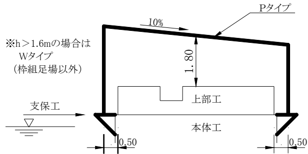
② 胸壁コンクリート（構造物高さ h > 1.6\text{m} 手摺先行型枠組足場を設置できる場合）
