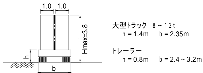
運搬車の積載方法の標準
