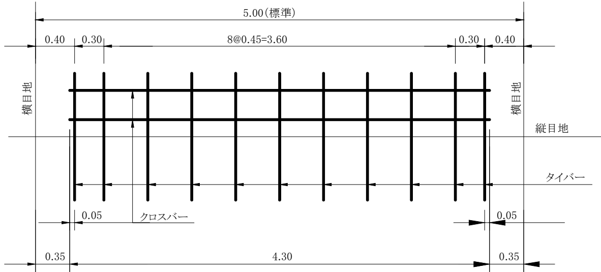
[平面図]
