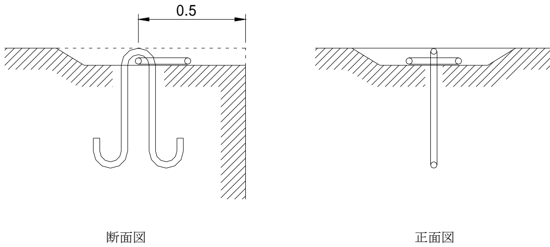
〔係船環配置例〕
