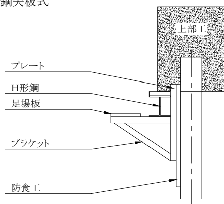
鋼矢板式
