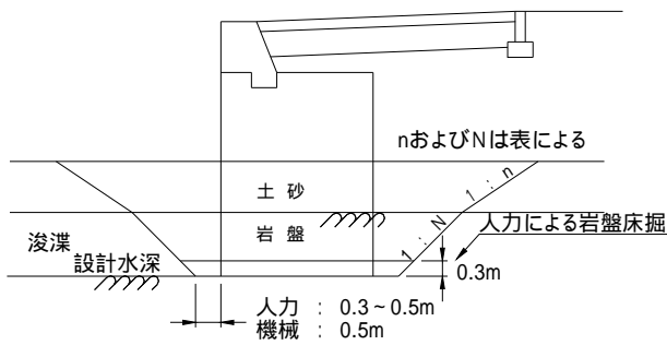
岩盤と土砂
