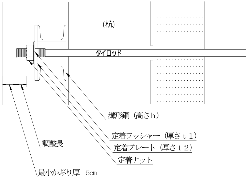
取付詳細図
