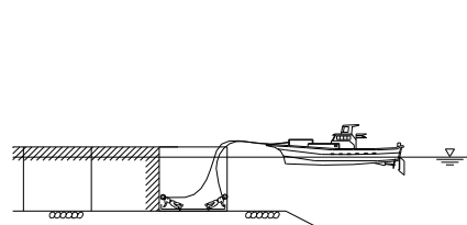
漏洩防止材
