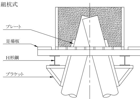
組杭式
