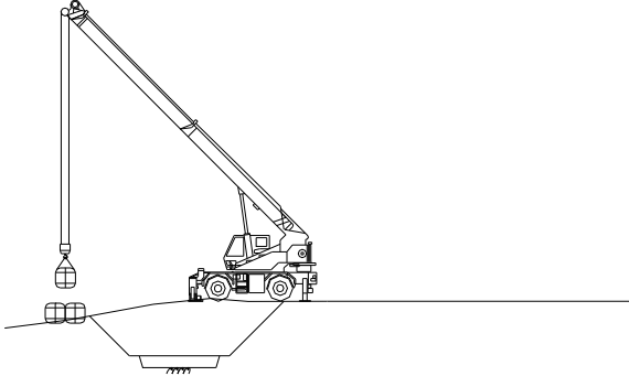
1) 仮設工 大型土のう据付
