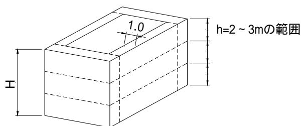
運搬可能なブロック状に分解する方法
