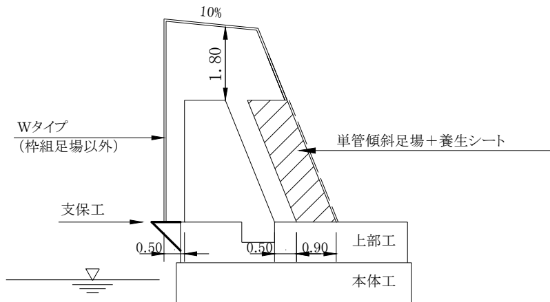
③ 胸壁コンクリート（構造物高さ h > 1.6\text{m} 手摺先行型枠組足場を設置できない場合）
