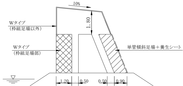
③ 胸壁コンクリート（構造物高さ h > 1.6\text{m} 手摺先行型枠組足場を設置できない場合）
