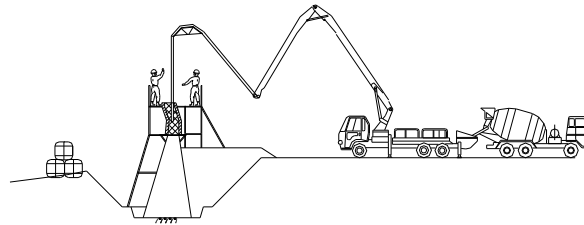
8) 波返工 場所打擁壁工 (構造物単位)
