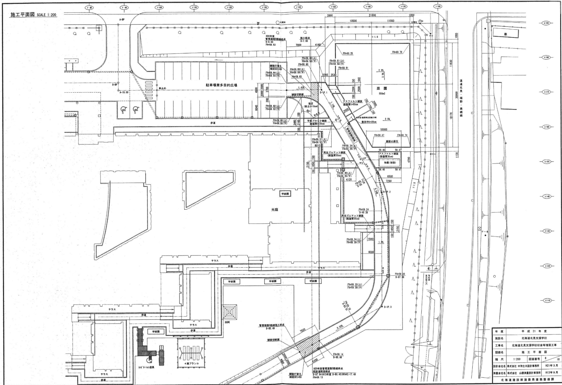
添付資料（7）外構施工平面図（北海道北見支援学校校舎等増築工事（平成22年1月竣工））
