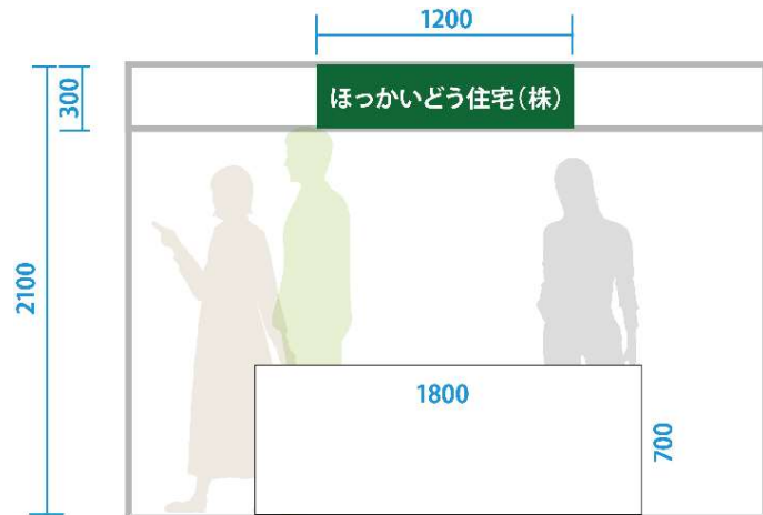
立面図
