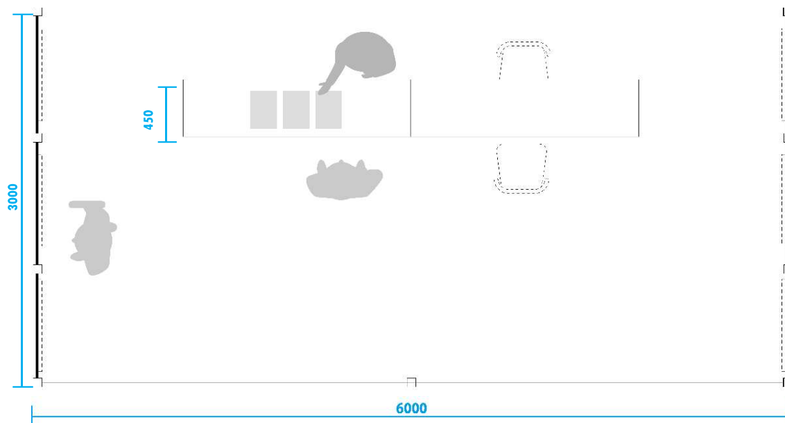
平面図
