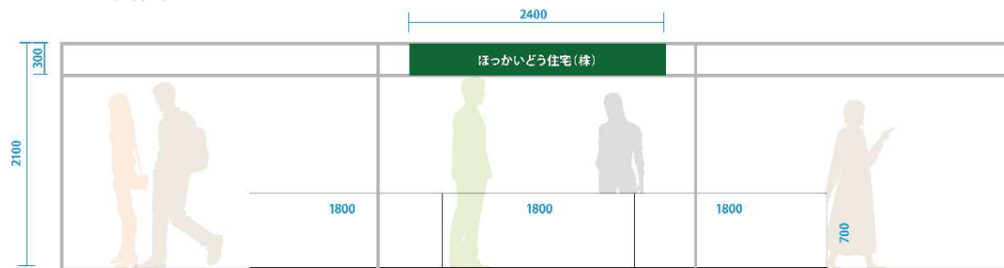
立面図
