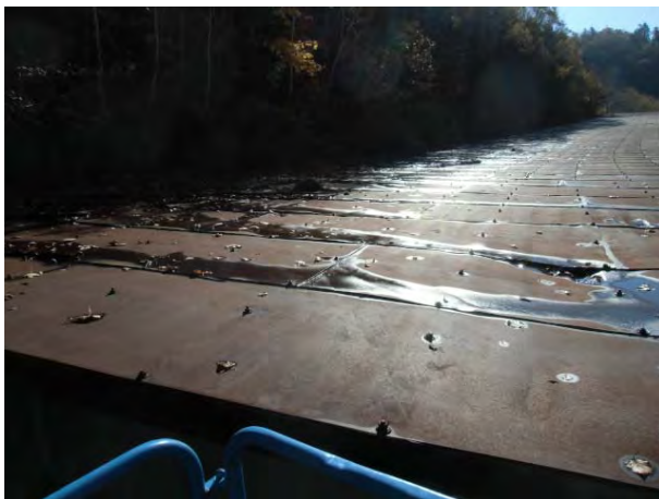
鋼製部材の変形例
