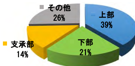
図 5-7 シェルターの変状等部位の状況
