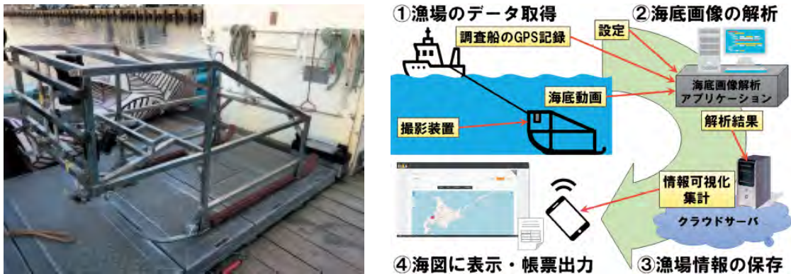
[図 3-9] けん引式撮影装置（左図）とホタテガイ漁場可視化システムの概要図（右図）
