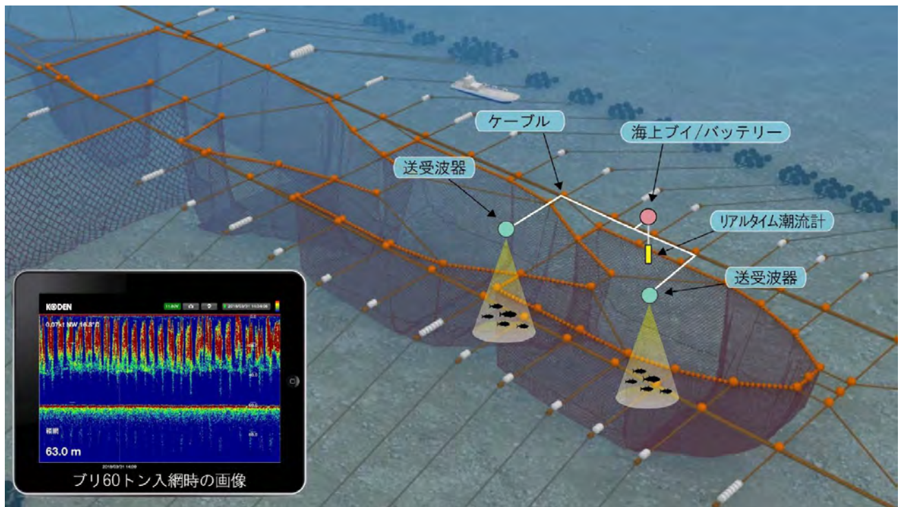
[図 3 - 3] 遠隔魚群探知機の稼働イメージ（提供：株式会社日東製網）
