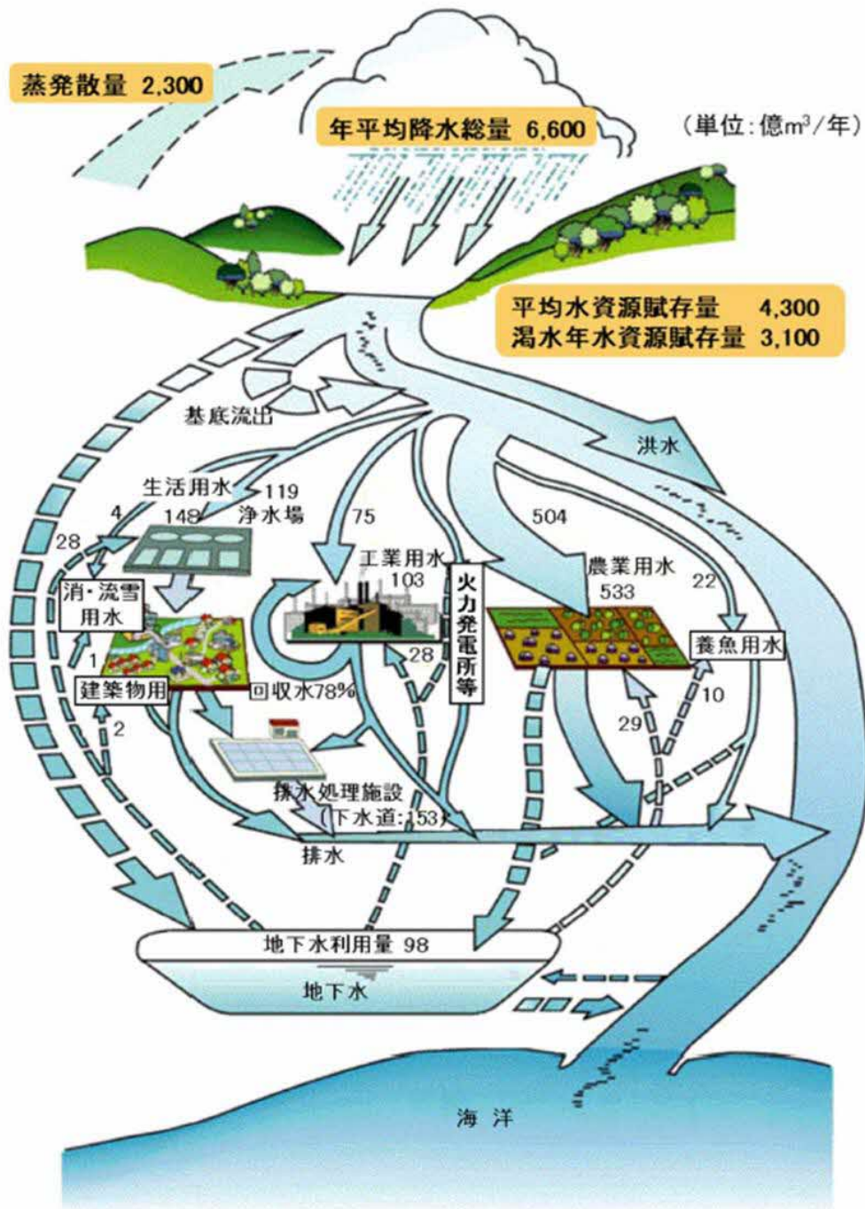
日本の水収支[参考:図1-2-1]
