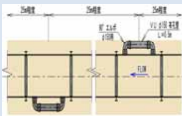
排水路の平面図
