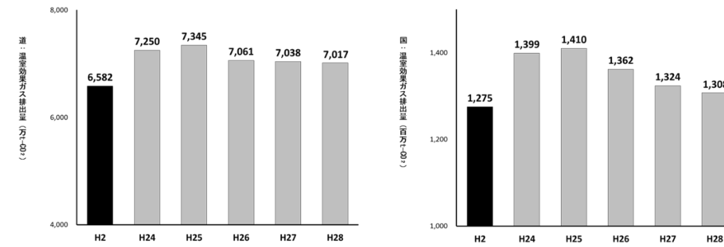
図2-1-1 北海道と全国の温室効果ガス排出量
