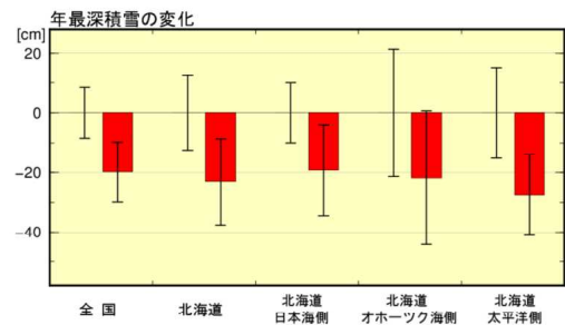
図4-17 全国および北海道の年最深積雪の変化 (単位: cm)
