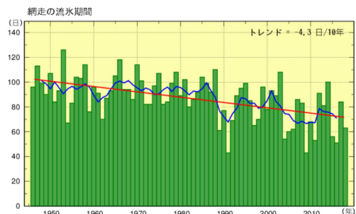
図4-7 網走における流氷期間の経年変化 (1946～2018年、単位：日)
