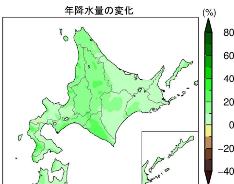
図4-13 北海道の年降水量の変化 (21世紀末の気候の20世紀末の気候に対する比、単位：%) 20世紀末気候に対する変化率で示す。緑系の色は増加、茶系の色は減少することを示す。
