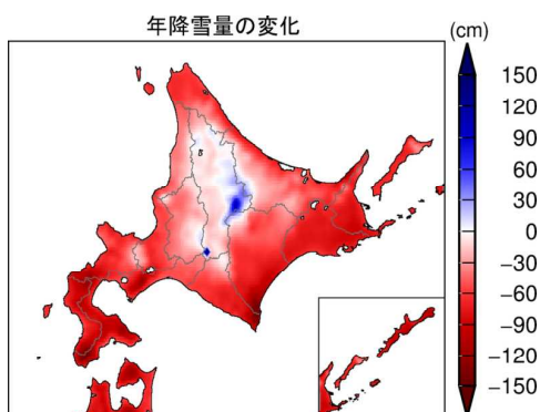
図4-18 年降雪量の変化 (単位: cm) 21世紀末の気候と20世紀末の気候との差を示す。
