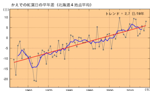
図4-9 北海道4地点（札幌、帯広、釧路、函館）を平均したかえでの紅葉日の経年変化（1953～2018年、単位：日）
