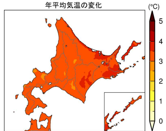
図4-10 北海道の年平均気温の変化（21世紀末の気候と20世紀末の気候との差、単位：℃）
