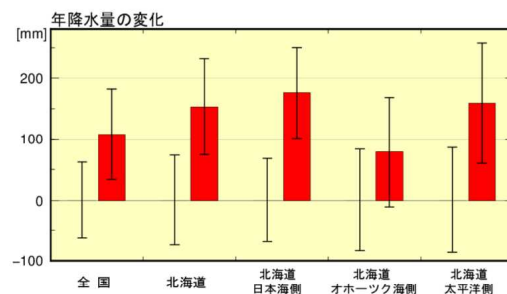
図4-14 全国および北海道の年降水量の変化 (単位：mm)
