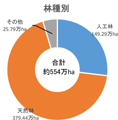
図3-3 森林面積
