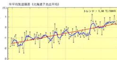
図4-1 北海道7地点（旭川、網走、札幌、帯広、根室、寿都、函館）を平均した年平均気温の経年変化（1898～2018年、単位：℃）
