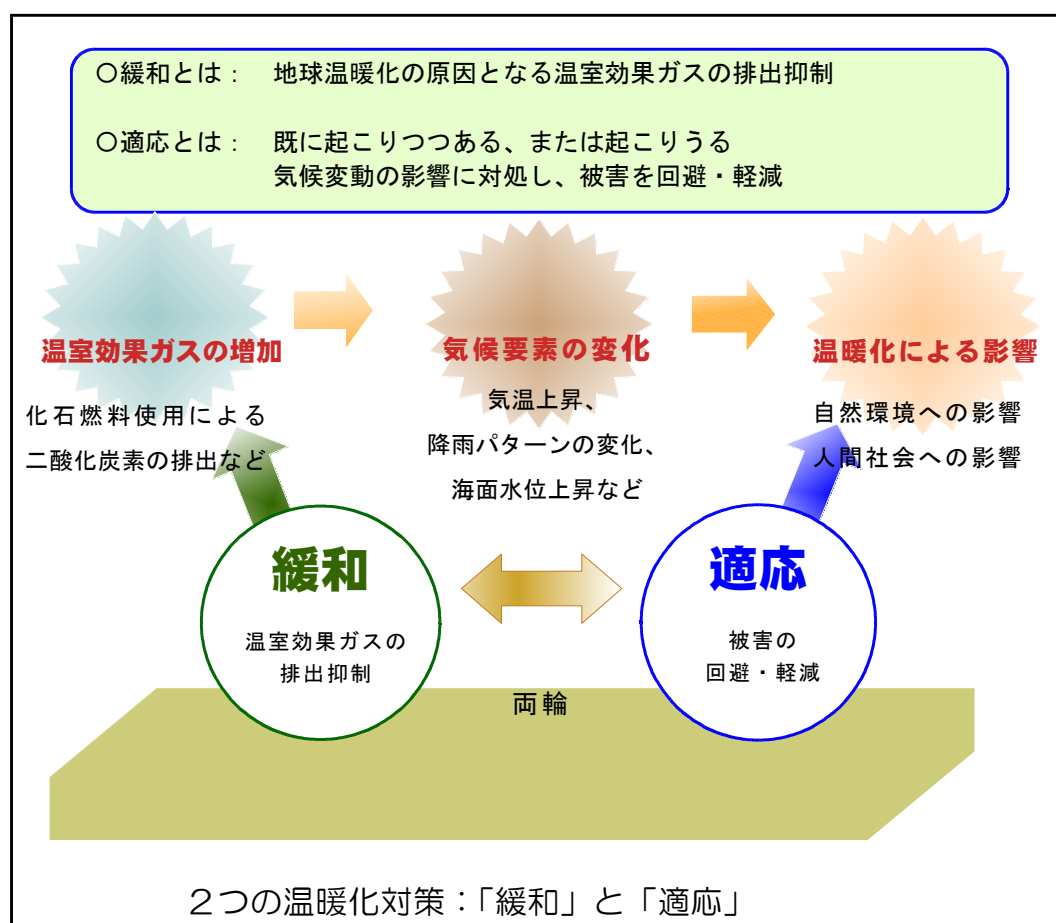
図1-1 「緩和」と「適応」
