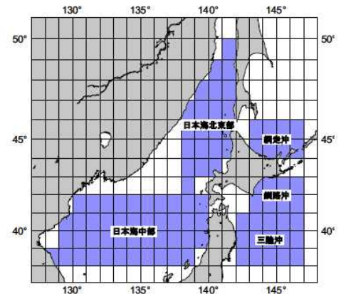
図4-5 海面水温の領域平均に用いた海域区分
