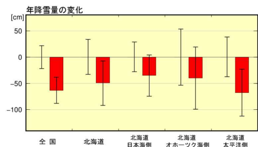
図4-19 全国および北海道の降雪量の変化 (単位: cm)
