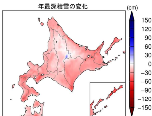
図4-16 年最深積雪の変化 (単位: cm) 21世紀末の気候と20世紀末の気候との差を示す。
