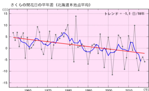
図4-8 北海道8地点（稚内、旭川、網走、札幌、帯広、釧路、室蘭、函館）を平均したさくらの開花日の経年変化（1953～2018年、単位：日）
