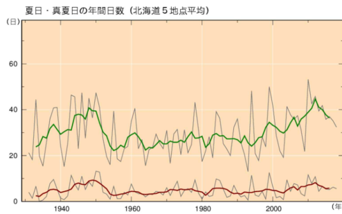
図4-2 北海道5地点（網走、札幌、帯広、根室、寿都）で平均した夏日、真夏日、冬日、真冬日の1地点あたり年間日数の経年変化（1931～2018年、単位：日） 左図は夏日（緑）、真夏日（茶）の経年変化を、右図は冬日（緑）および真冬日（青）の経年変化をそれぞれ示す。細線は各年の値を、太線は5年移動平均をそれぞれ示し、直線（赤）は期間にわたる変化傾向を示す。なお、真夏日の日数は夏日の日数に、真冬日の日数は冬日の日数にそれぞれ含まれる。
