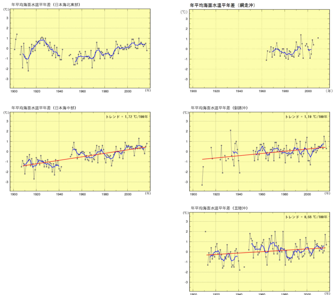
図4-6 各海域における年平均海面水温の経年変化 (単位: °C)
