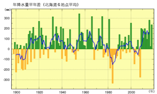
図4-3 北海道6地点（旭川、網走、札幌、帯広、根室、寿都）を平均した年降水量の経年変化（1898～2018年、単位：mm） 棒グラフは各観測地点での年降水量の基準値からの偏差を平均した値を示している。青線は偏差の5年移動平均を示す。基準値は1981～2010年の30年平均値。
