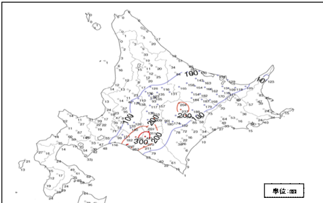
図 - 2 総雨量分布図（8月17日0時～19日9時）
