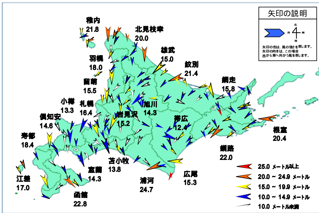
図 - 3 最大風速分布図 (1月7日0時～9日0時)
