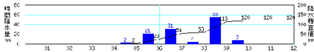
図 - 4 1時間雨量と積算雨量の時系列 (7月28日0時～12時)
