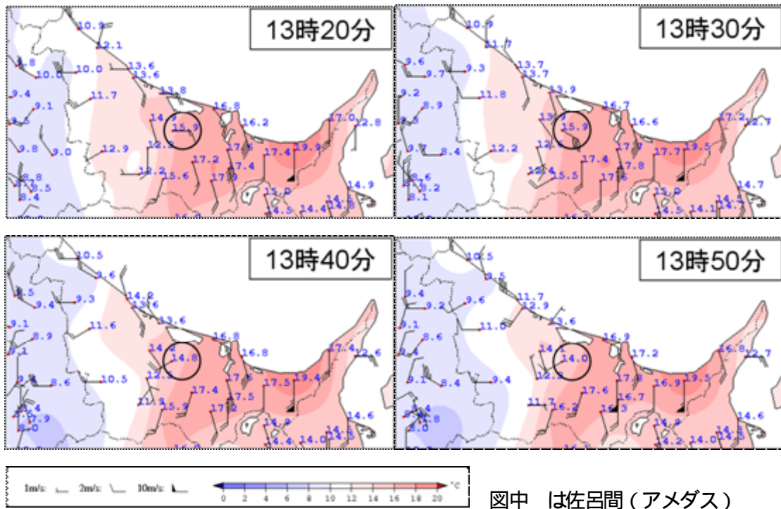
図 - 3 アメダスの気温と風の分布 (11月7日13時20分～13時50分)
