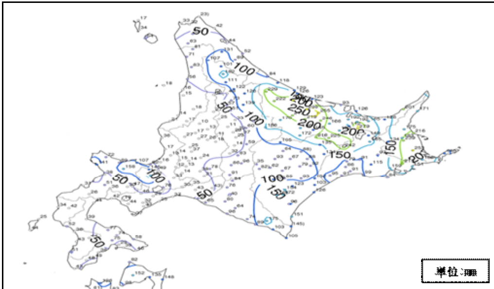
図 - 2 総雨量分布図（10月6日0時～10日0時）
