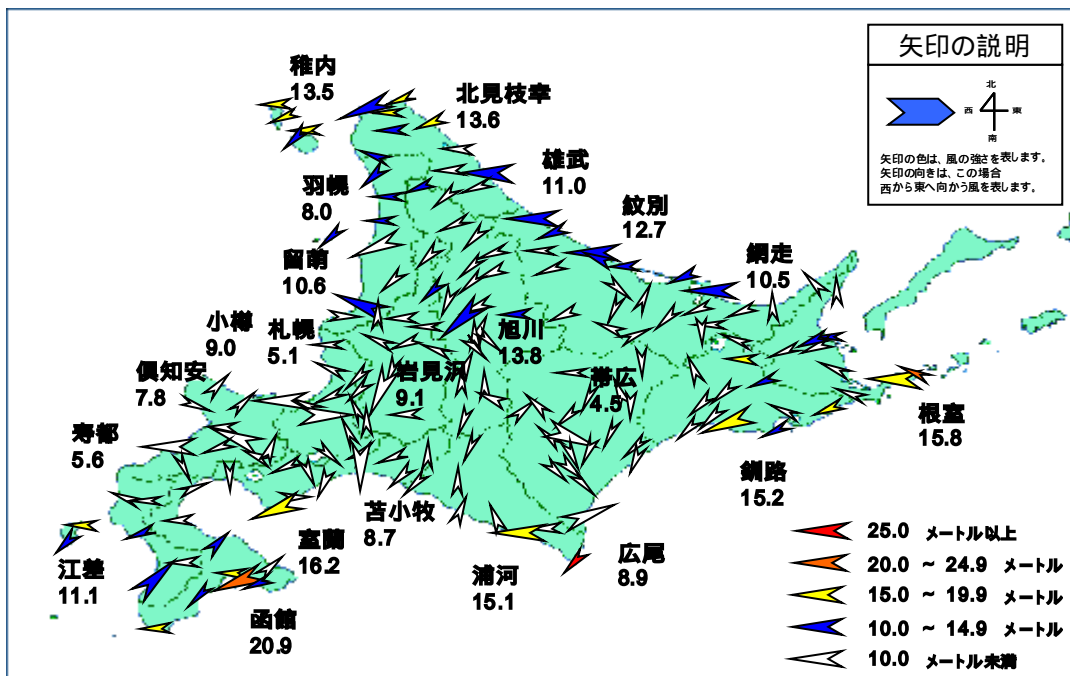
図 - 3 最大風速分布図 (9月7日0時～9日0時)
