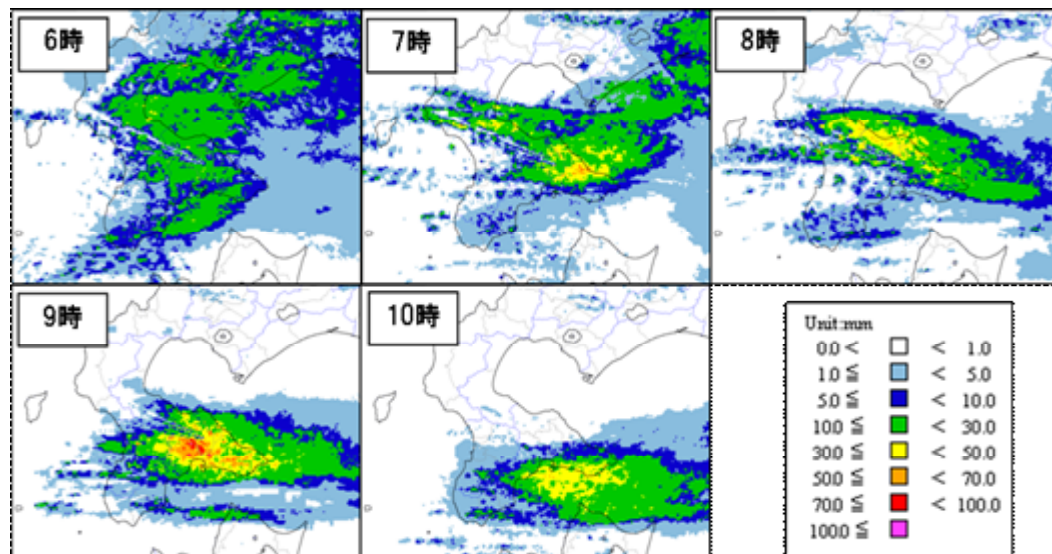
図 - 2 解析雨量図(7月28日6時~10時)
