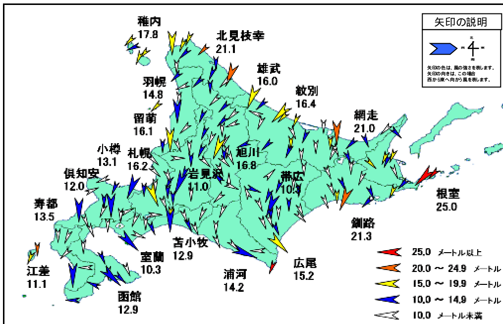
図 - 3 最大風速分布図（10月6日0時～10日0時）
