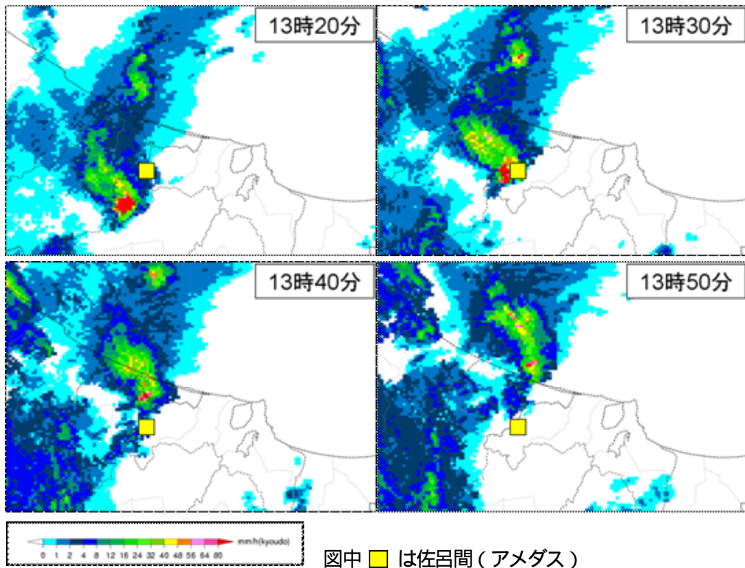
図 - 4 レーダーによる雨雲の動き (11月7日13時20分～13時50分)
