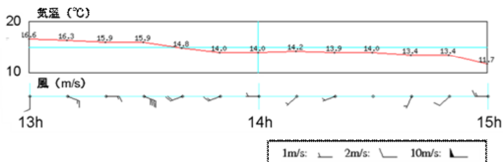
図 - 2 佐呂間 (アメダス) の気温と風の時系列 (11月7日13時00分～15時00分)
