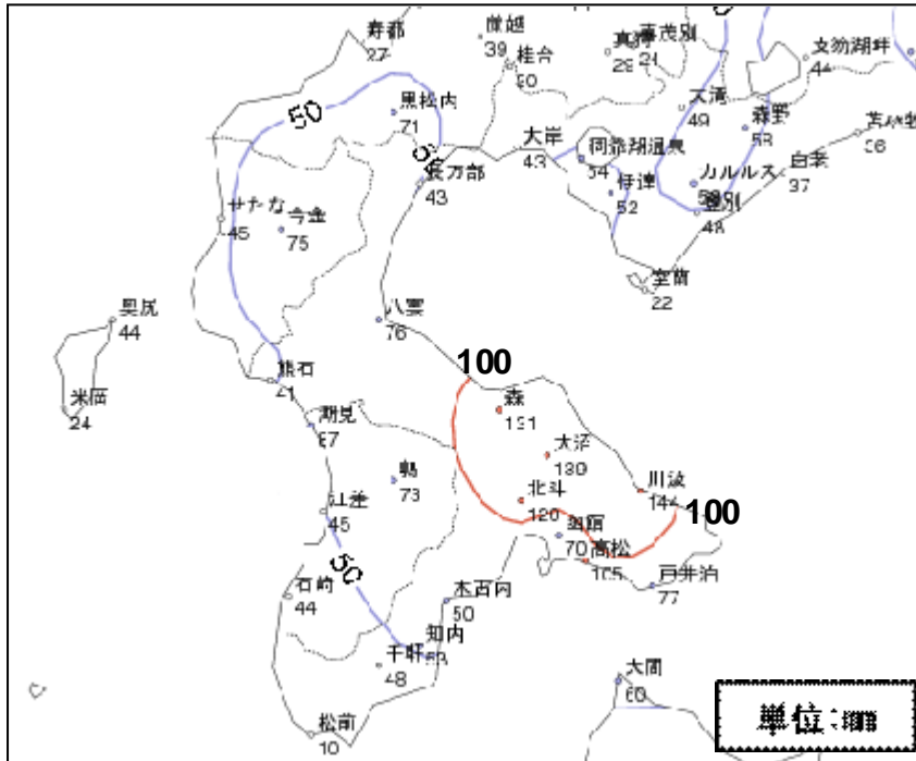
図 - 3 総雨量分布図 (7月28日0時～12時)
