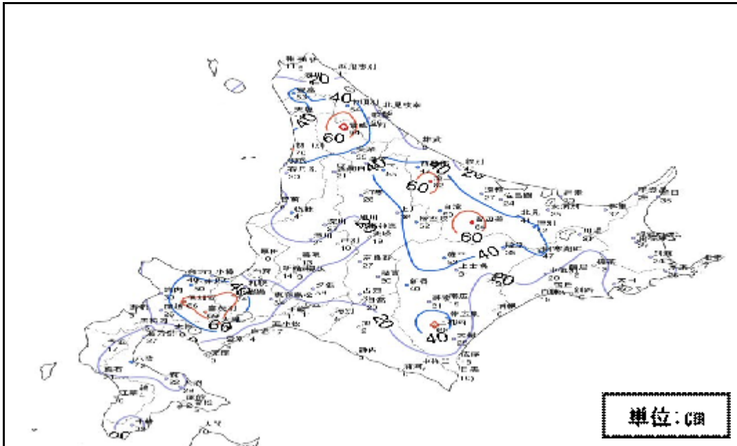
図 - 2 総降雪量分布図 (1月6日9時～9日9時)
