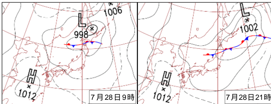
図 - 1 地上天気図
