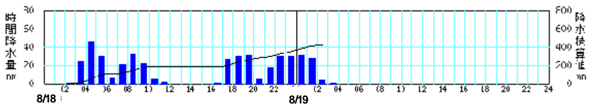
図 - 3 1時間雨量と積算雨量の時系列（8月18日0時～20日0時）
