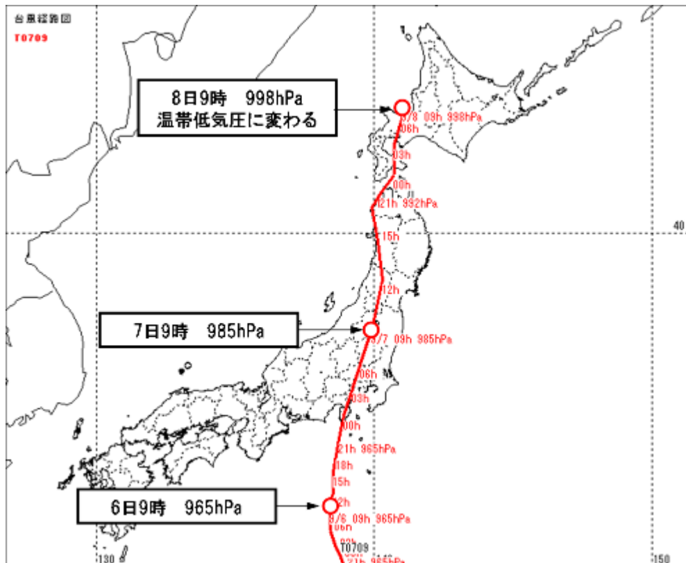
図 - 1 台風第9号の経路図
