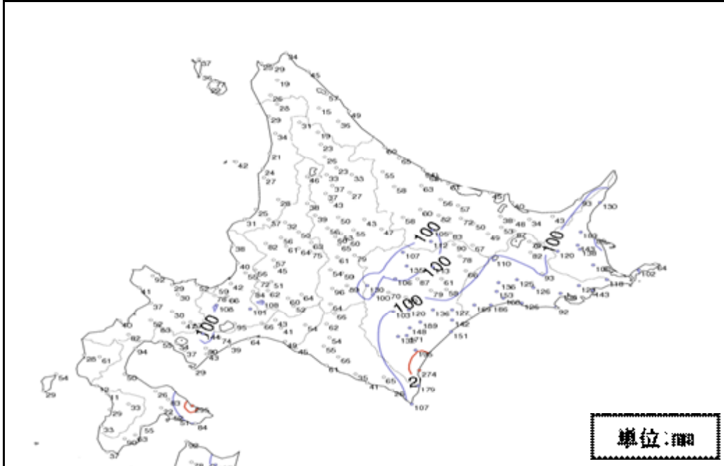
図 - 2 総雨量分布図 (9月6日8時～8日15時)
