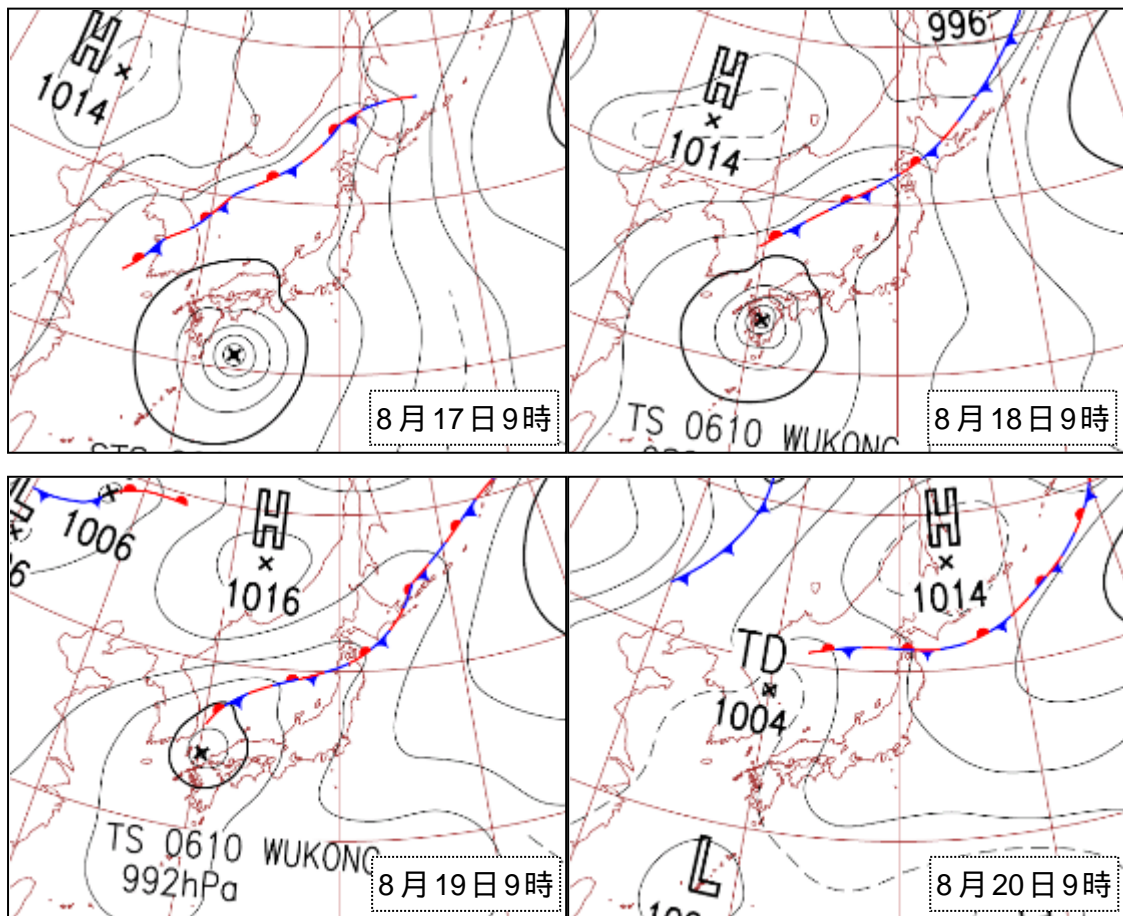
図 - 1 地上天気図
