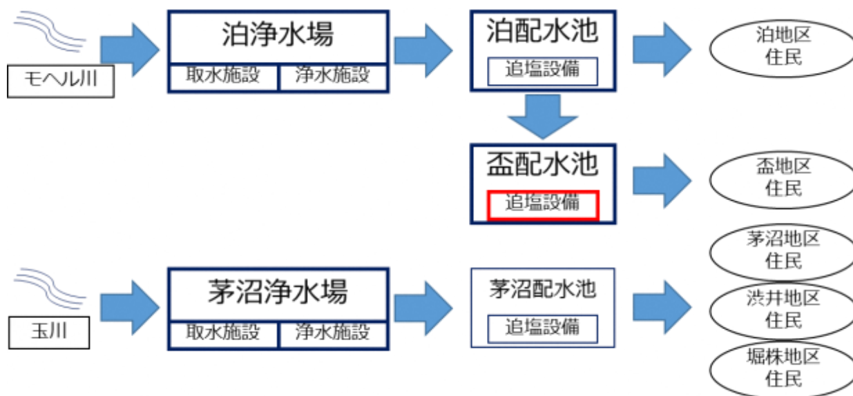
泊村簡易水道施設系統図
