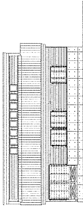
東立面図
