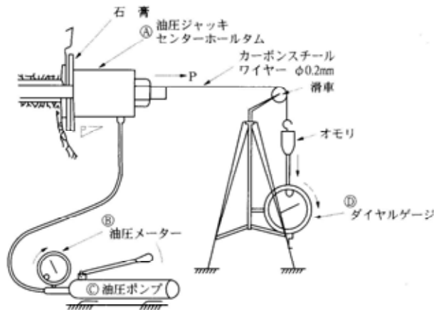
図－３ 引抜試験概要図
