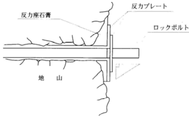
図－２ 反力座の設置
