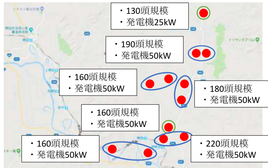
(3)問寒別地区個別型&共同型バイオガスプラントモデル(12戸)
