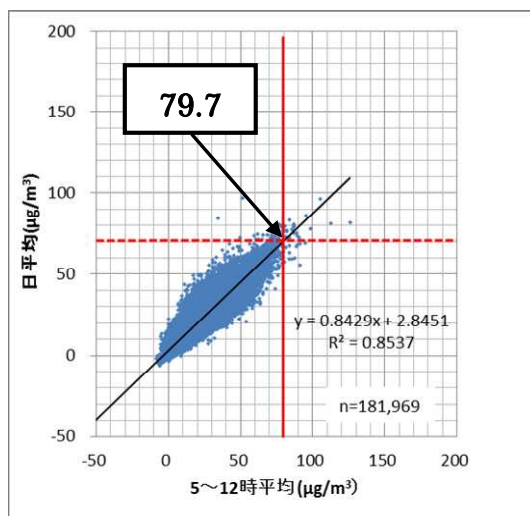
図3 . 日平均値と当該日の午前5時～午後12時の1時間値の平均値との回帰分析結果
