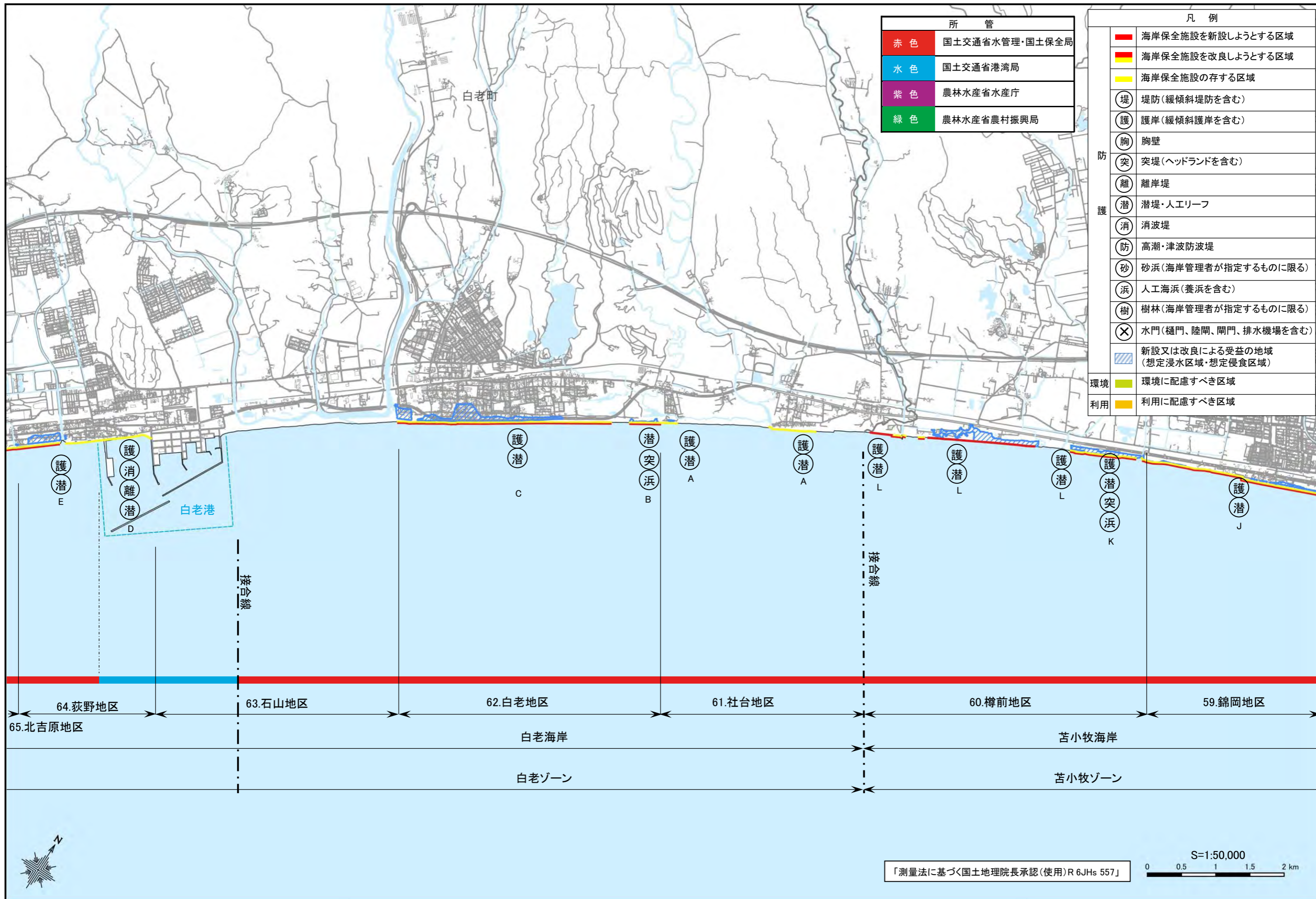
白老ゾーン 図面番号 1/2
