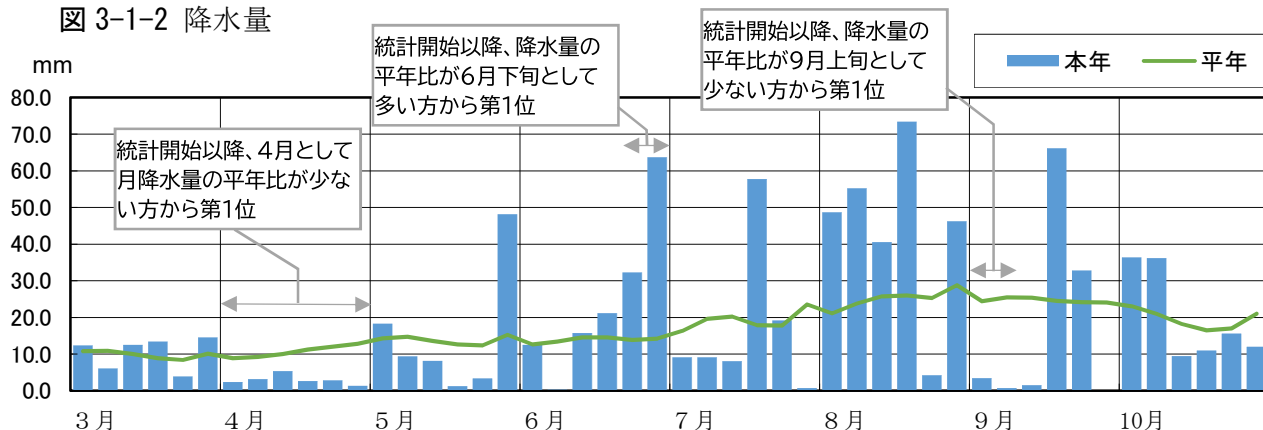
図 3-1-2 降水量
