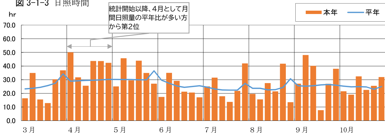
図 3-1-3 日照時間
