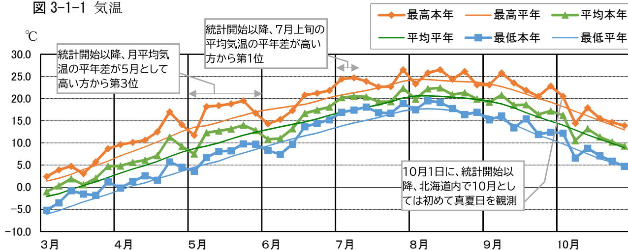
図 3-1-1 気温
