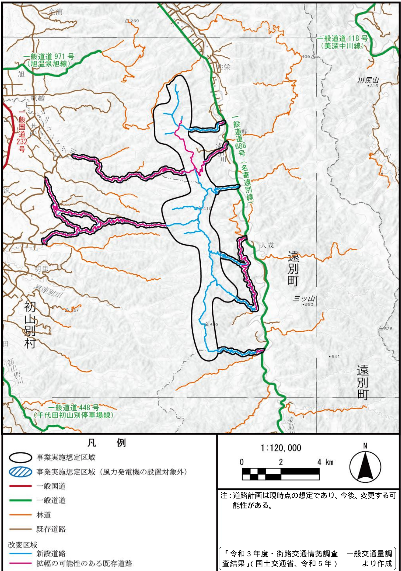
図1 道路計画
