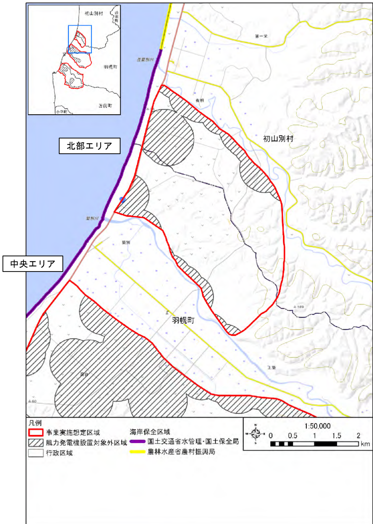
図 海岸保全区域の分布状況(詳細)(4/4)
