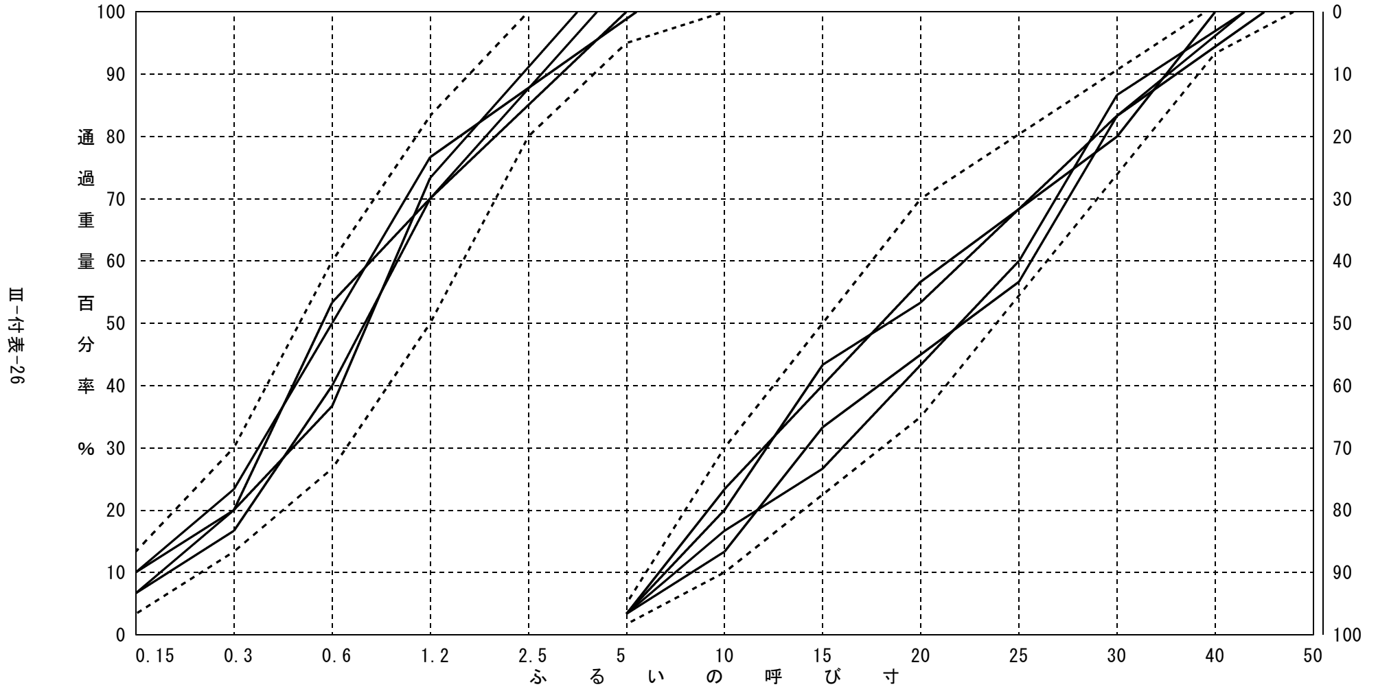
コンクリート骨材ふるい分け試験取りまとめ図（記載例）
