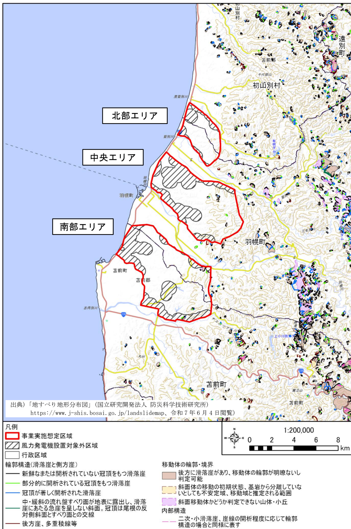
図 地すべり地形の分布状況
