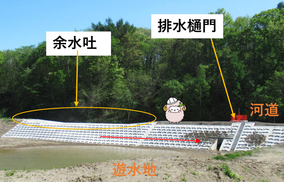
越流堤
