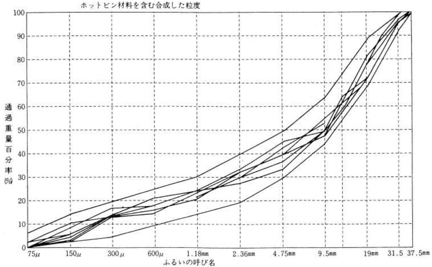
ふるい分け試験取りまとめ図 (記載例)
