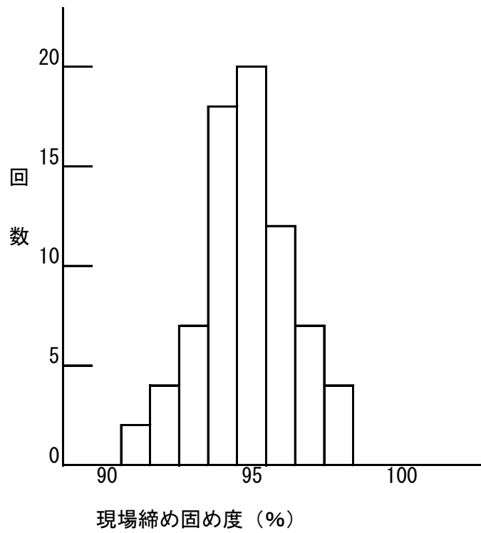
現場密度
