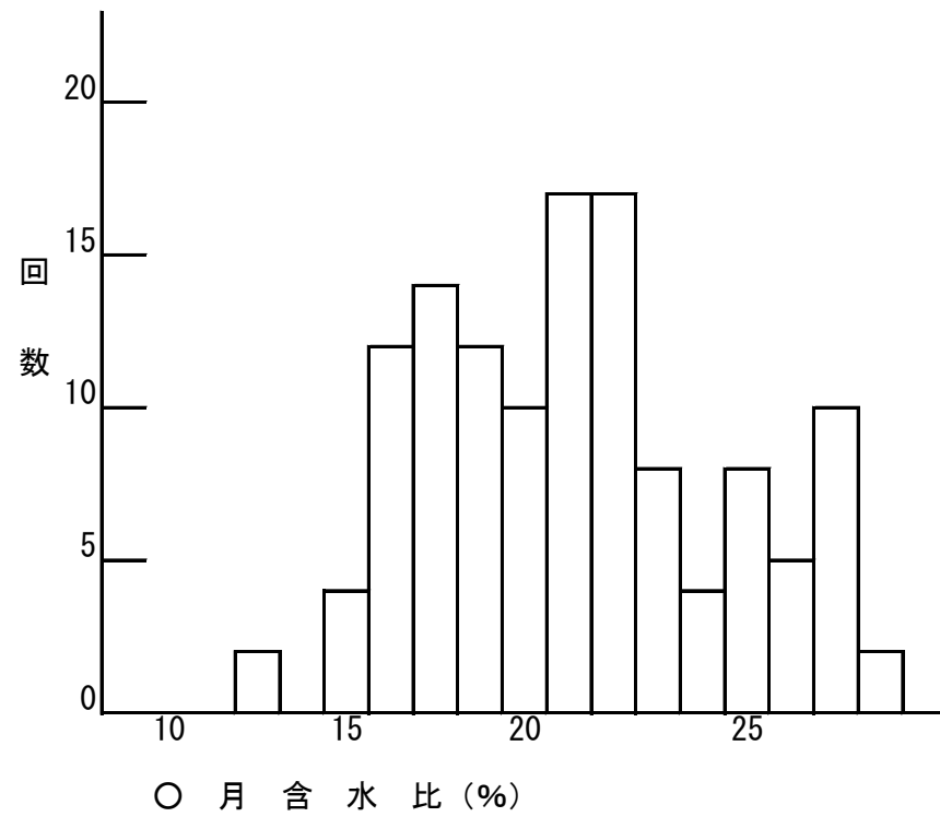
締め固め時の含水比
