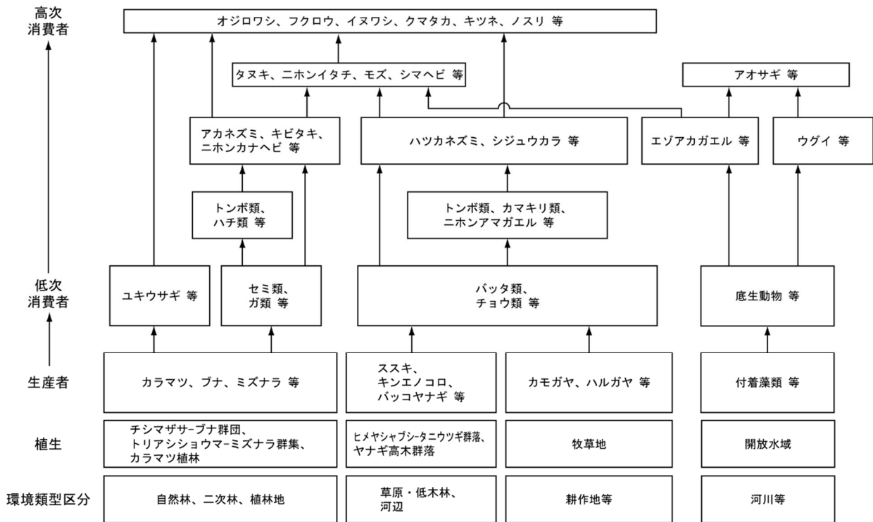
図 3.1-30 食物連鎖模式図
