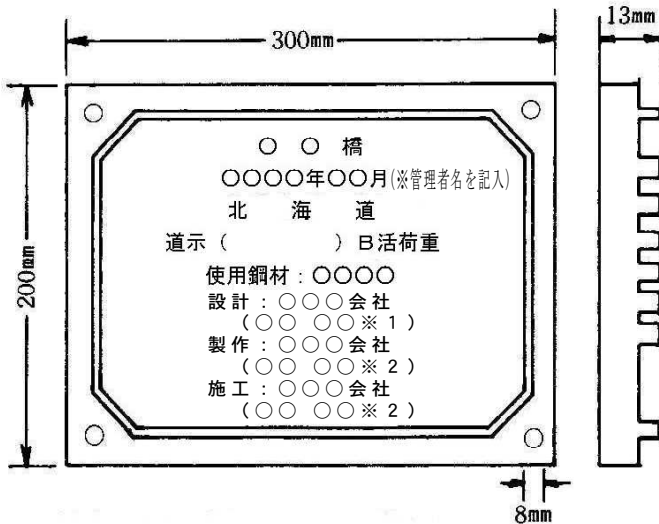
板厚8mm 字厚5mm 計13mm ※1 管理技術者氏名、※2 監理技術者氏名
