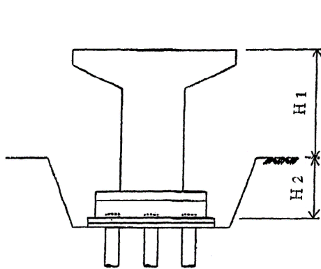
設置高さ = H1 + H2
