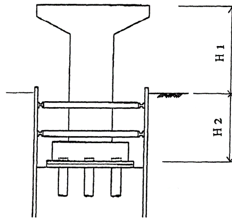
設置高さ = H1 + H2
