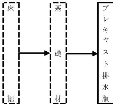
図2.1 施工フロー
