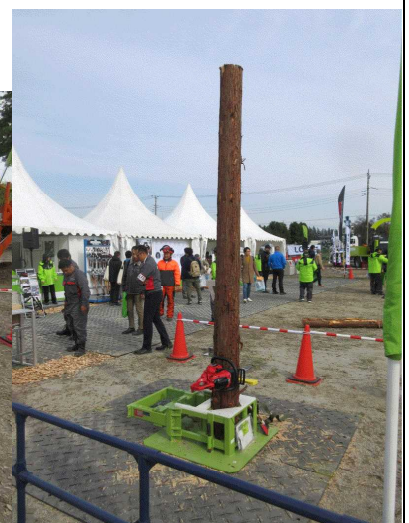
伐倒練習用丸太固定装置
