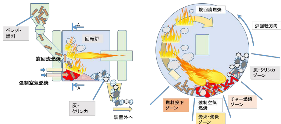
燃焼機内の構造、燃焼メカニズム
