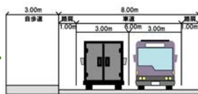
計画断面図
