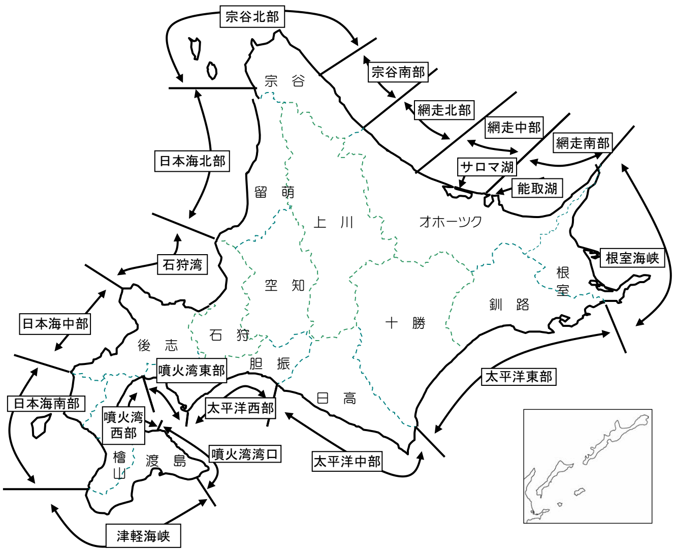
図6-5-1 平成29年度貝毒発生状況(ホタテガイ規制海域)
