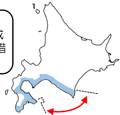
〈えりも以西海域の状況〉 (北海道水産現勢参照)
