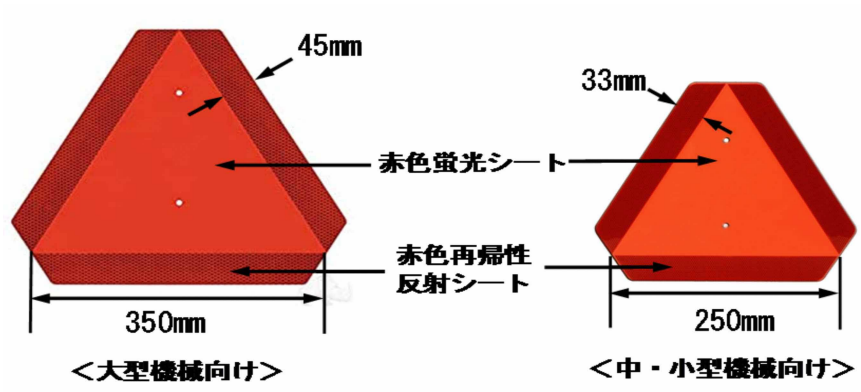
図11 低速車マーク ECE規格R69 住友3M社カタログより引用
