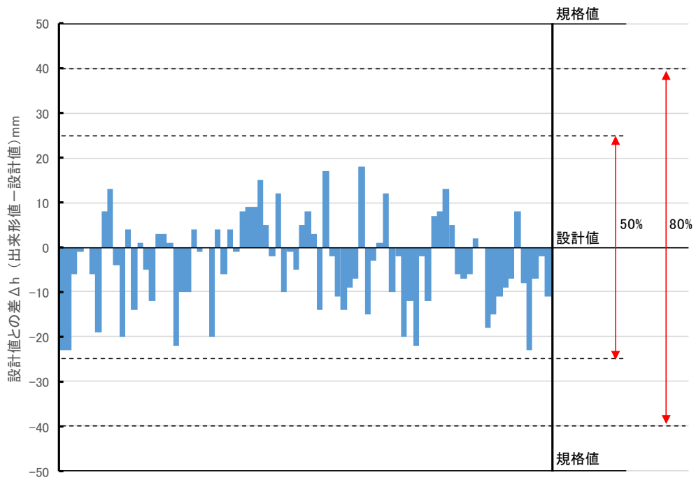
図 芽室北第3地区 14-2 圃場・設計値との差 ( \Delta h )
