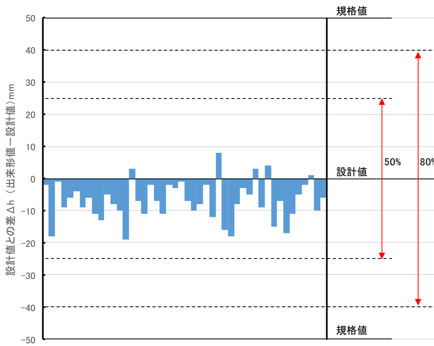
図 芽室北第3地区 21-1 圃場・設計値との差 ( \Delta h )
