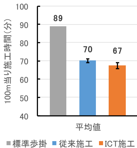
暗渠排水 バックホウ掘削 (スリムバケット)
