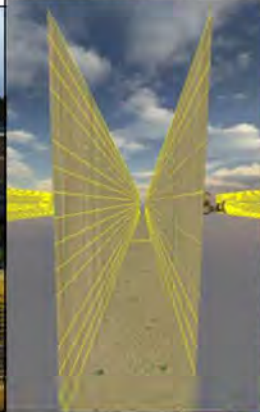
吸水渠断面の3D施工データ
