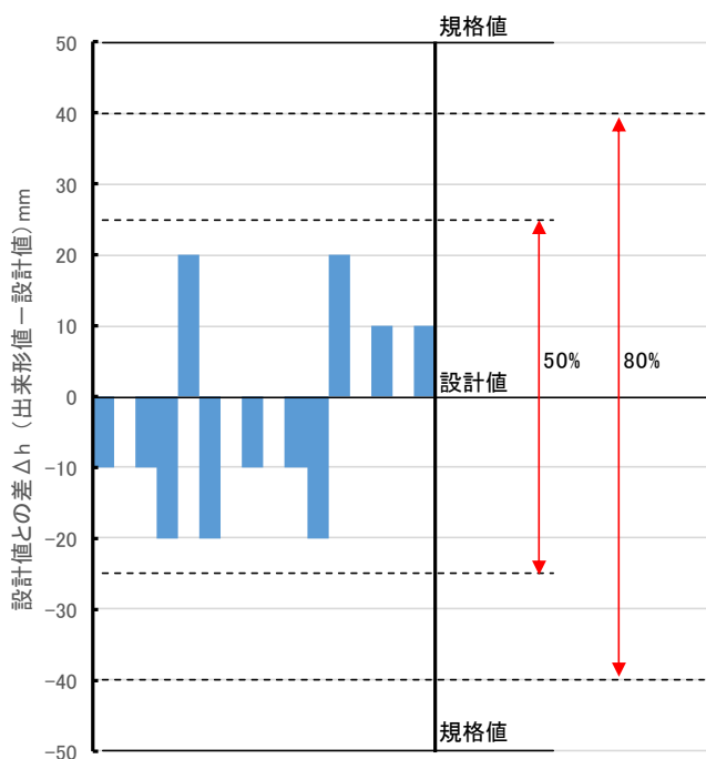
図 北見北地区・設計値との差 (Δh)
