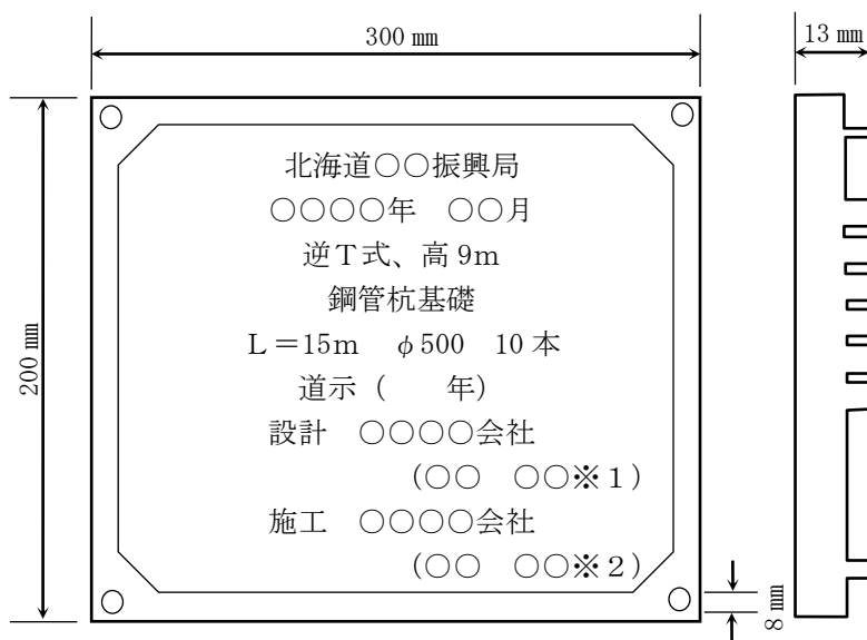
図 11-8-1 橋歴板
