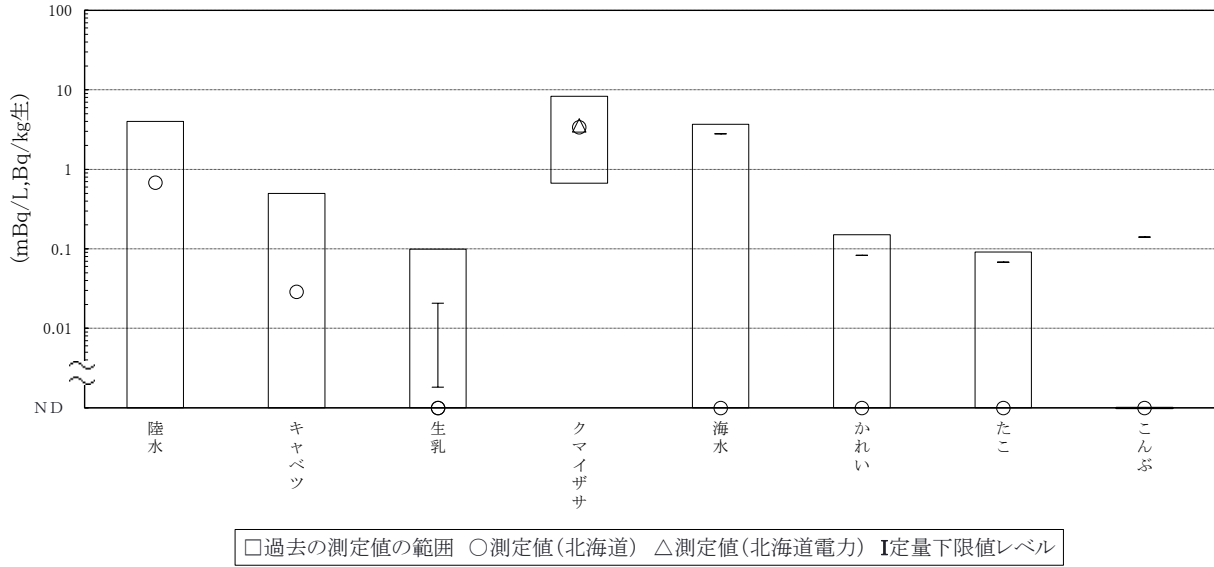
図3 ストロンチウム-90 分析結果
