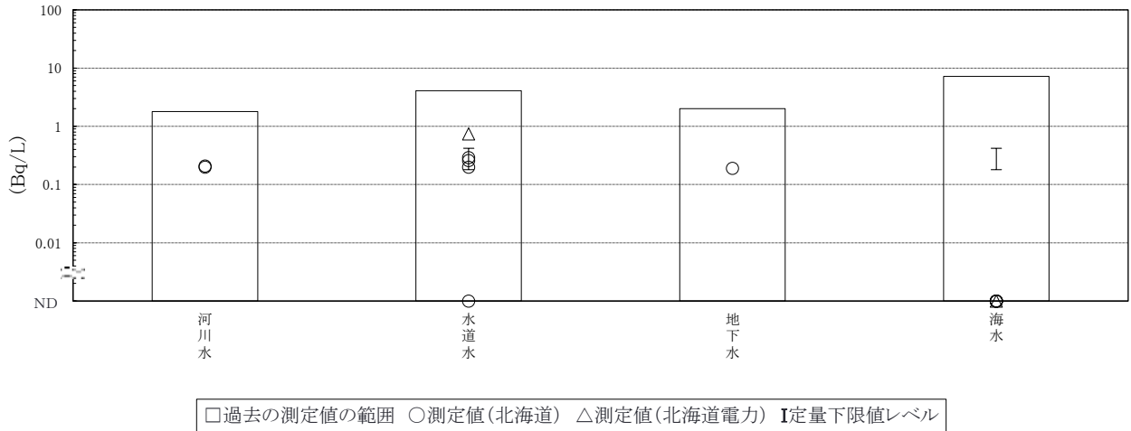
図4 トリチウム分析結果
