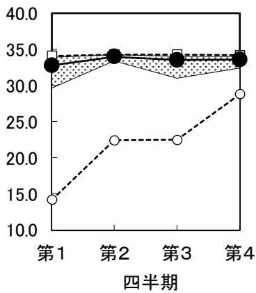
図3-1 塩分
