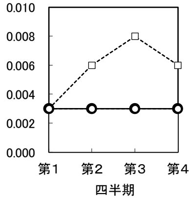
図3-11 NO 2 -N(mg/L)
