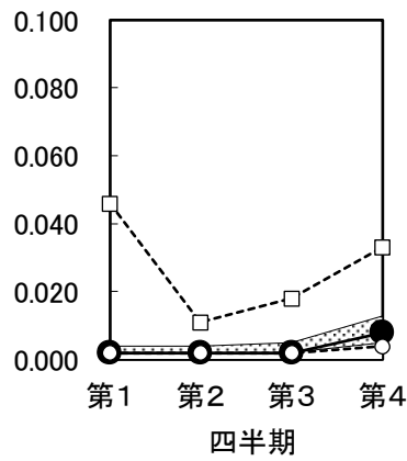
図3-8 PO 4 -P(mg/L)
