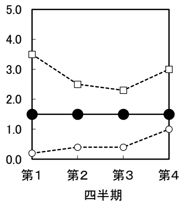
図4-2 透明度(m)
