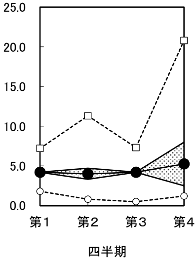
図5-5 COD(mg/g乾泥)
