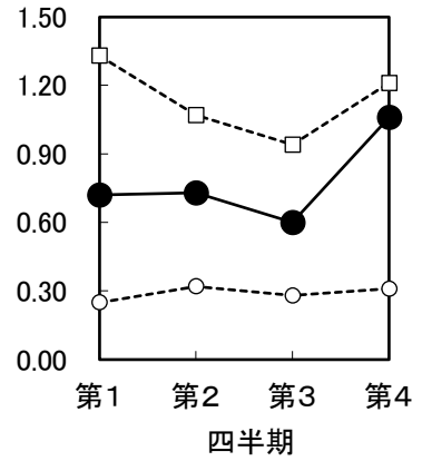
図4-9 T-N(mg/L)
