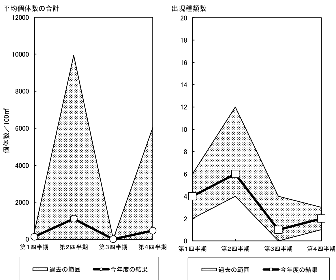
図 10-1 卵(MTD)
