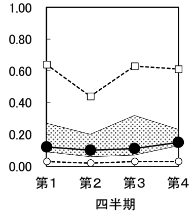
図3-9 T-N(mg/L)
