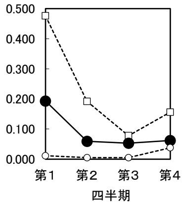
図4-10 NH 4 -N(mg/L)
