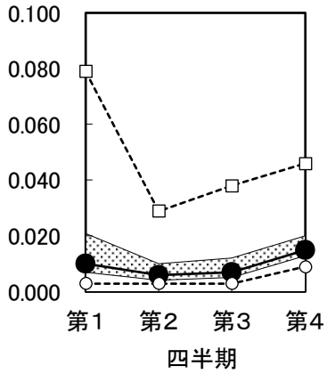
図3-7 T-P(mg/L)
