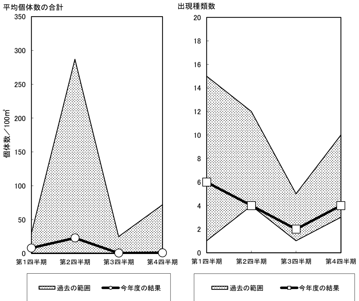
図 10-2 稚仔(MTD)
