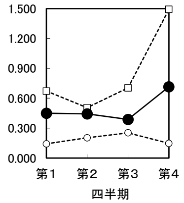
図4-12 NO 3 -N(mg/L)
