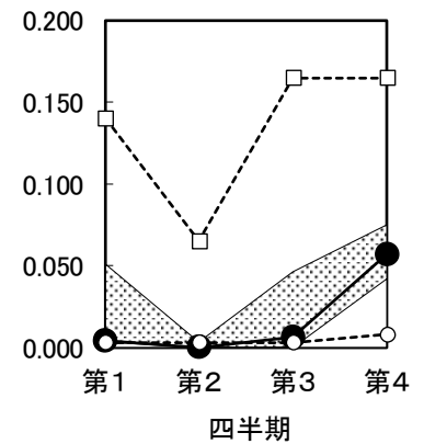
図3-12 NO 3 -N(mg/L)
