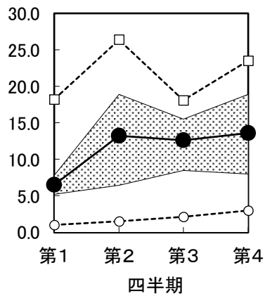
図3-2 透明度(m)
