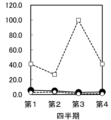
図4-6 SS(mg/L)
