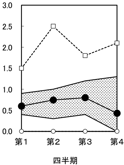
図5-1 COD(mg/g乾泥)
