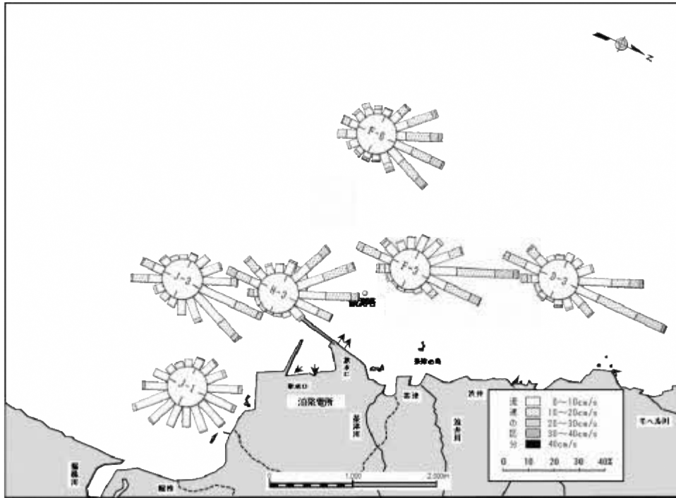
図 2-3 流向流速頻度分布図 (第 3 四半期)
