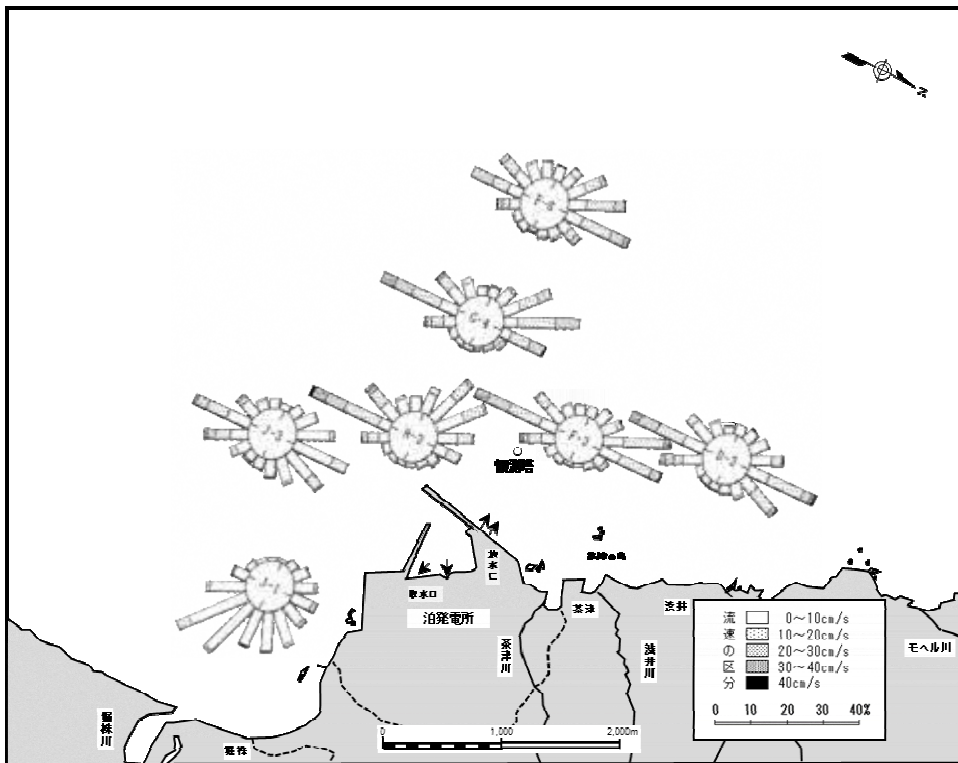
図 2-4 流向流速頻度分布図 (第 4 四半期)
