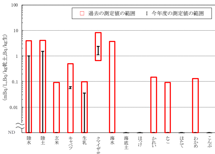
図2 ストロンチウム-90分析結果
