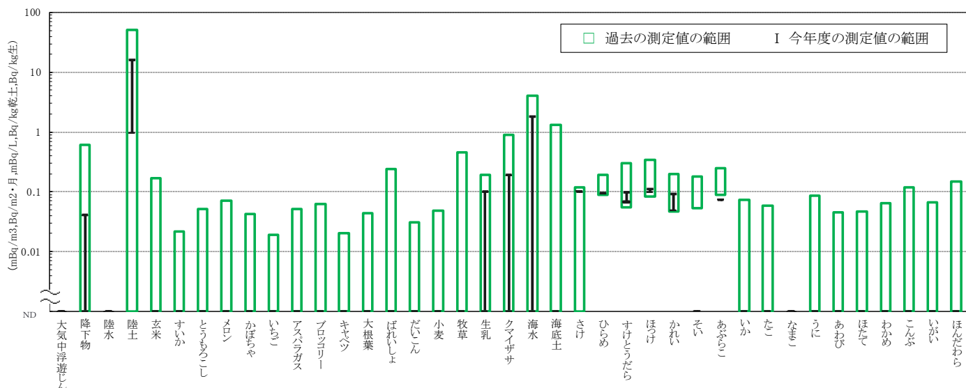
図2 ストロンチウム-90分析結果
