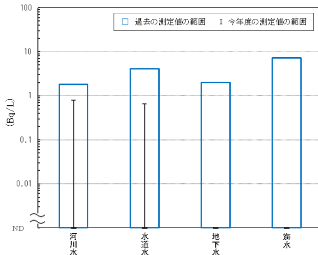
図3 トリチウム分析結果
