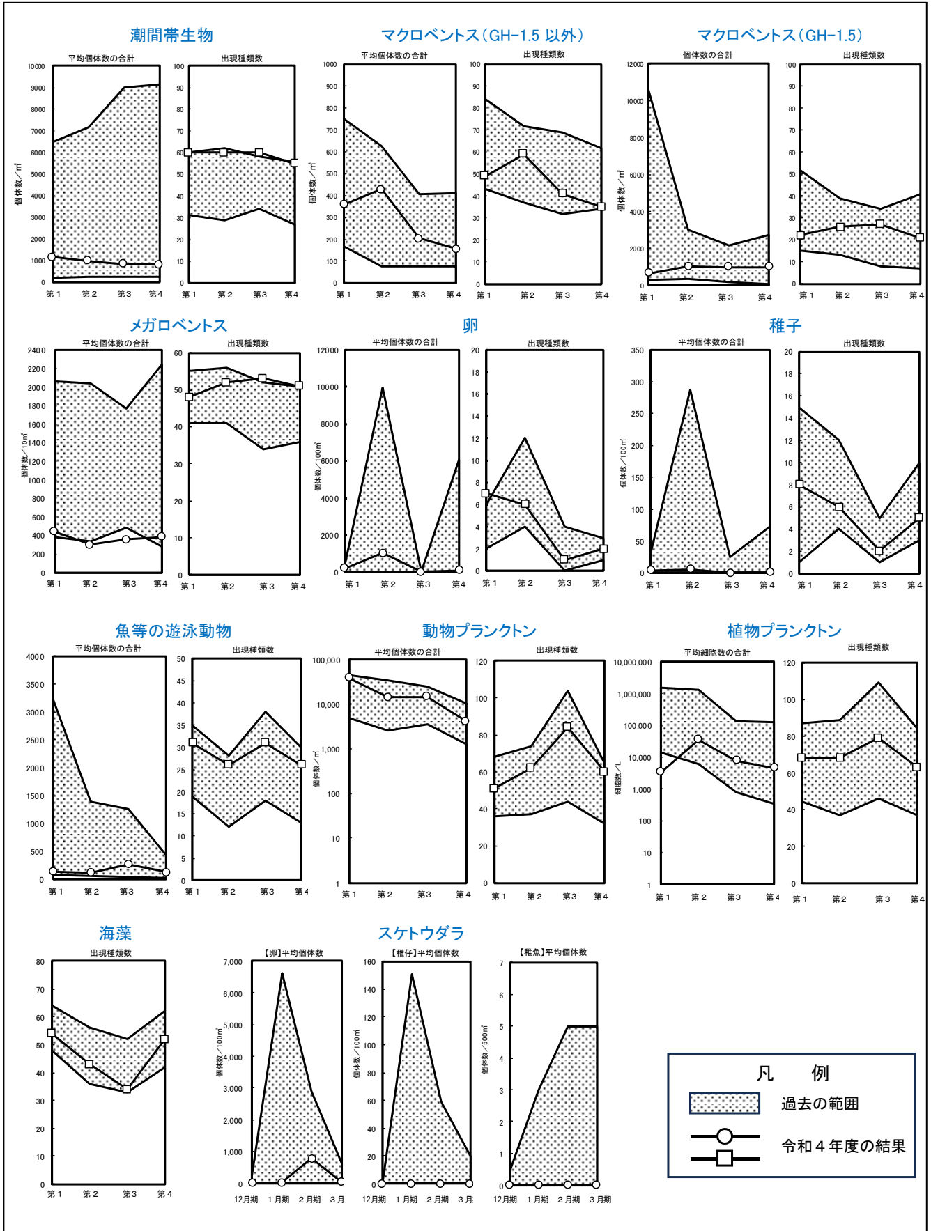
図7 海生生物調査結果
