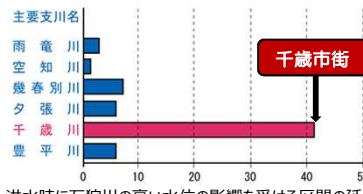
洪水時に石狩川の高い水位の影響を受ける区間の延長
