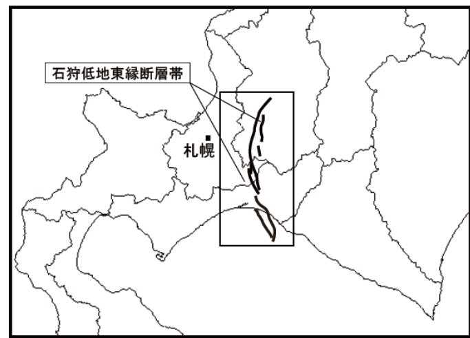
石狩低地東縁断層帯の位置
