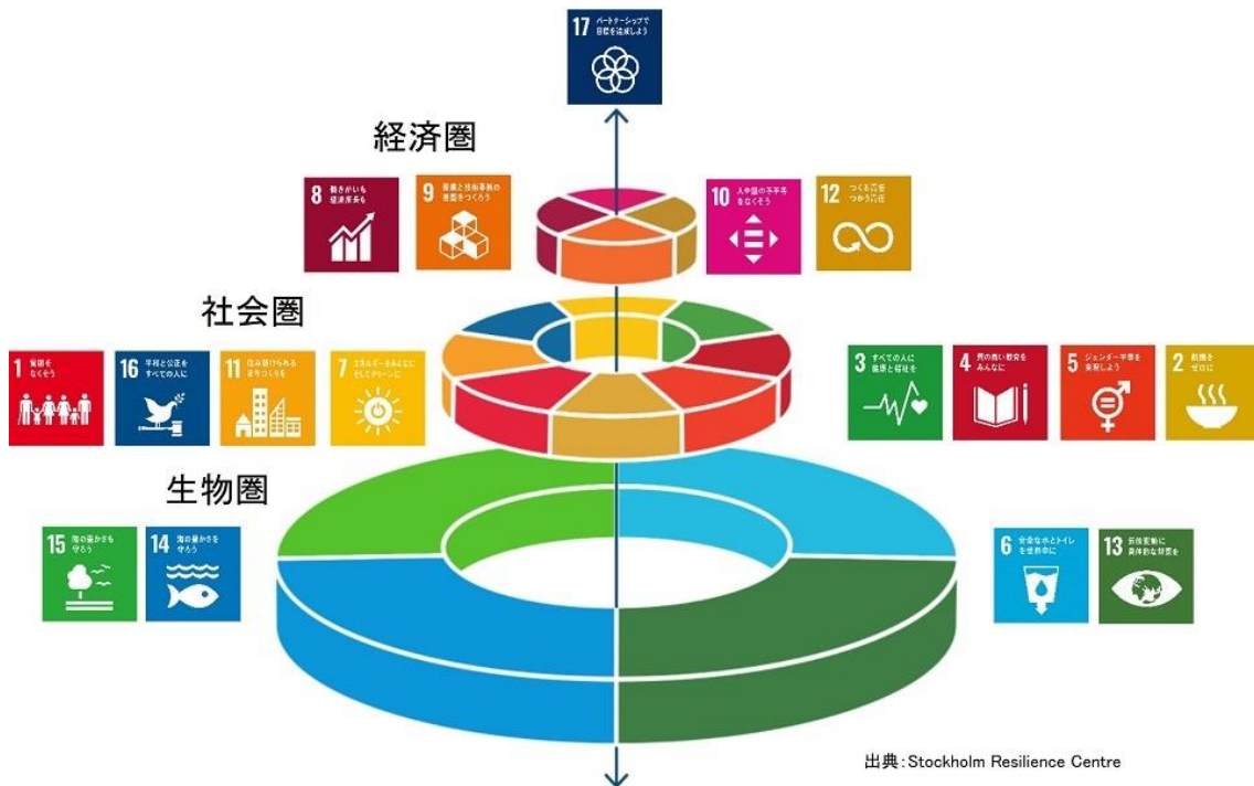
14 図 SDGsウェディングケーキ図
