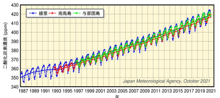
図 気象庁の観測点における二酸化炭素濃度の経年変化
